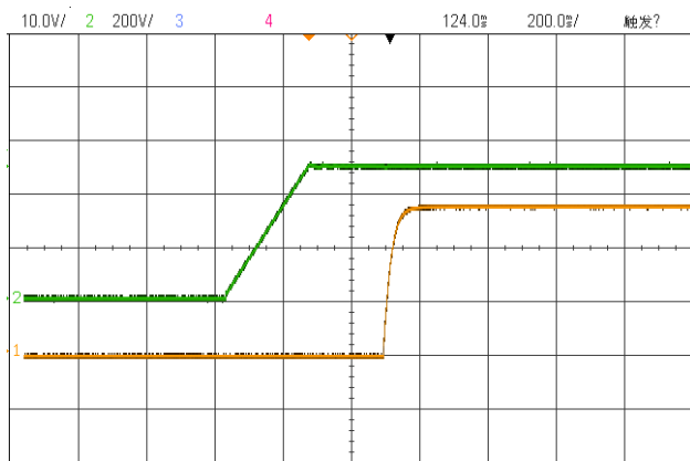
启动波形(额定输入, 满载) CH1:输出电压 CH2:输入电压
