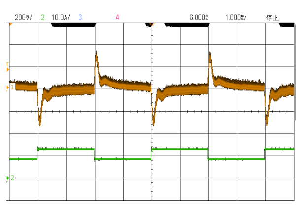
输出电压动态波形 (额定输入, 75%~50%~75% Io)
