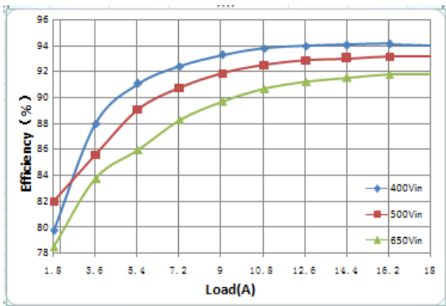
效率曲线
