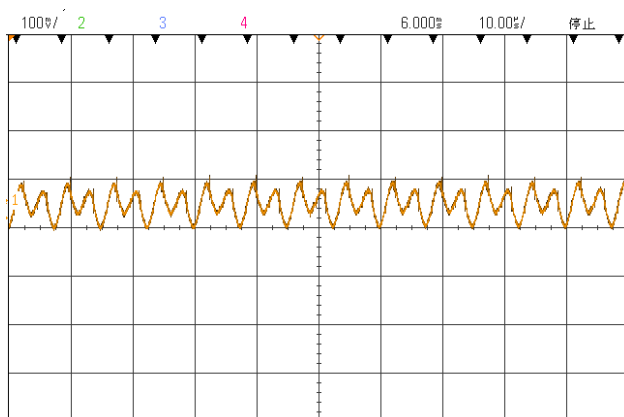
输出纹波电压波形(额定输入, 满载)
