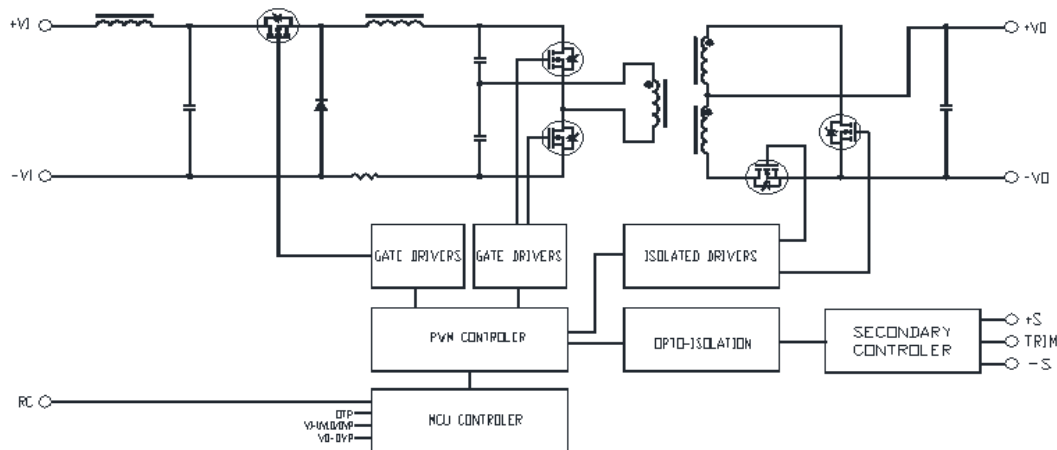
模块功能框图
