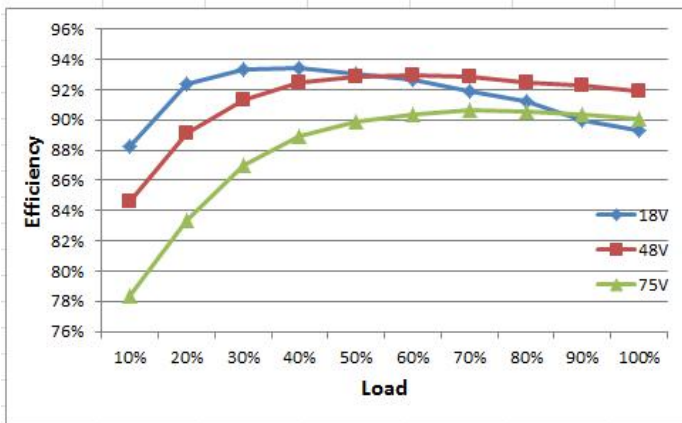
效率曲线
