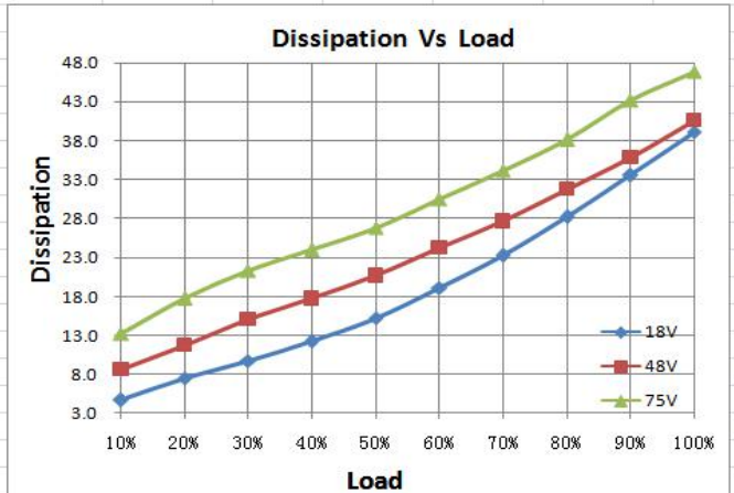
损耗曲线
