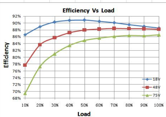
效率曲线
