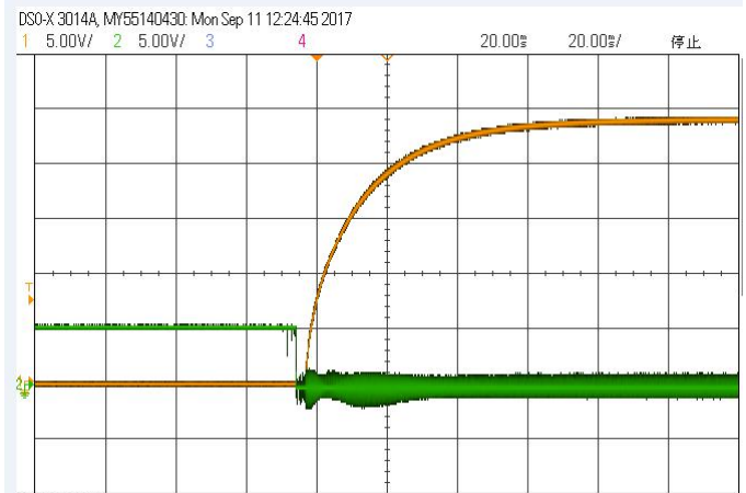
使能起机波形 (负逻辑)
