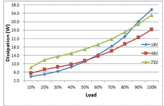
损耗曲线
