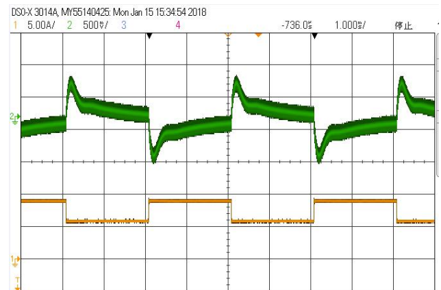
输出电压动态波形 (50%~75%~50%Iout)
