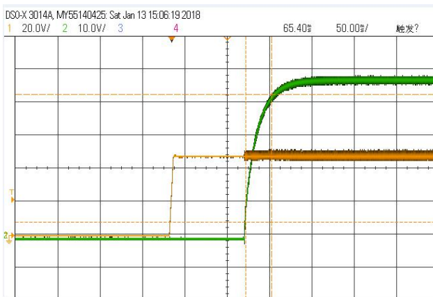
启动波形(额定输入,满载)
