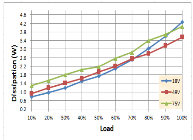
损耗曲线
