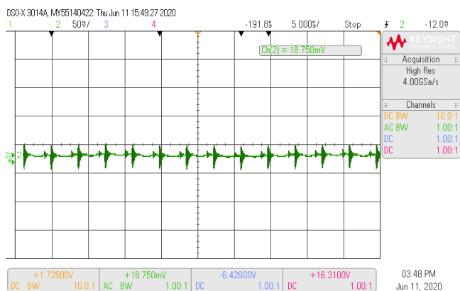
纹波(额定输入,满载)
