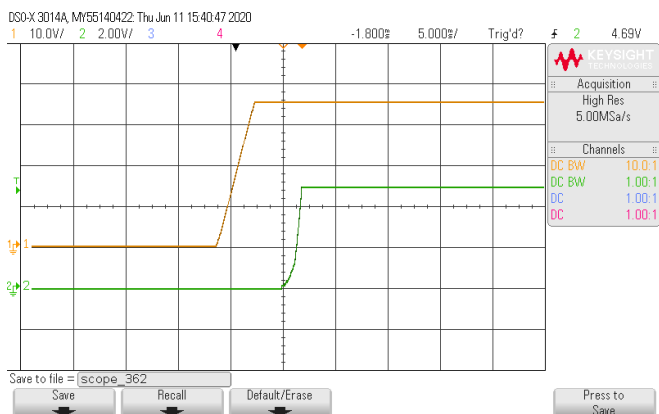
启动波形(额定输入,满载)
