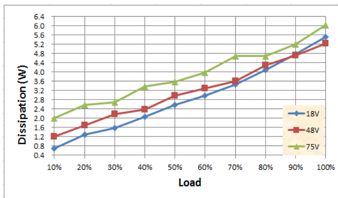
功率损失
