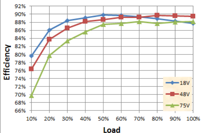
效率曲线
