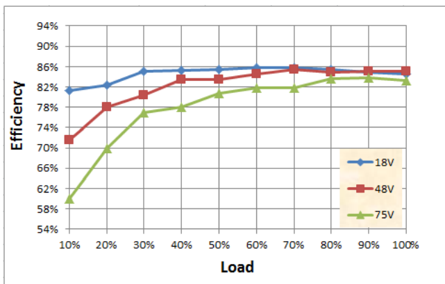
效率曲线
