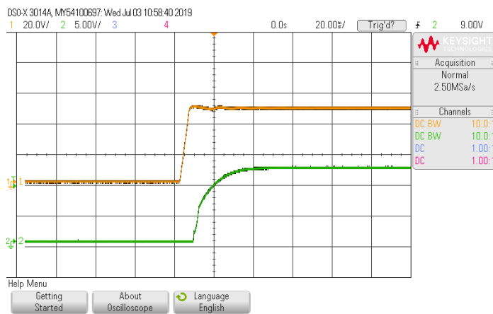
启动波形(额定输入,满载)
