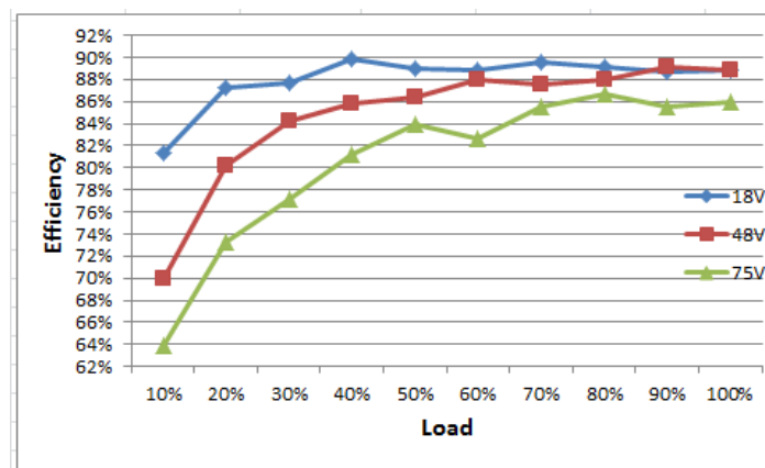
效率曲线
