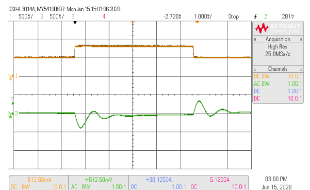
动态波形 (75%~50%~75% Iout)
