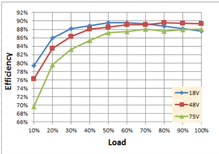
效率曲线
