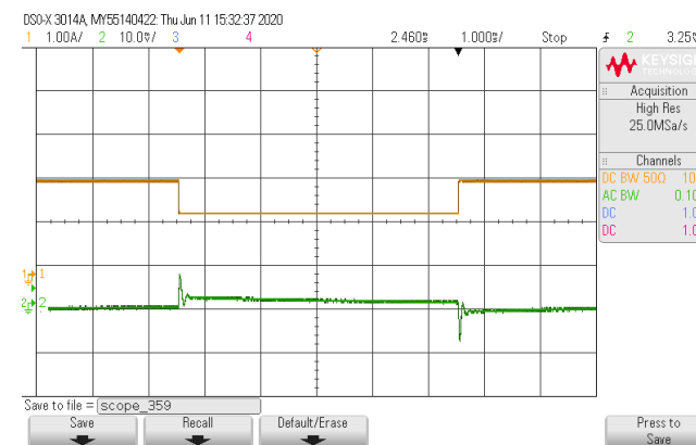
输出电压动态波形 (75%~50%~75% Iout)
