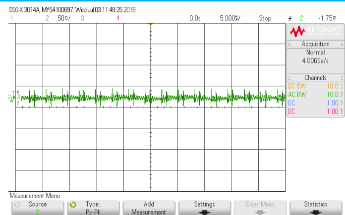
纹波(额定输入,满载)
