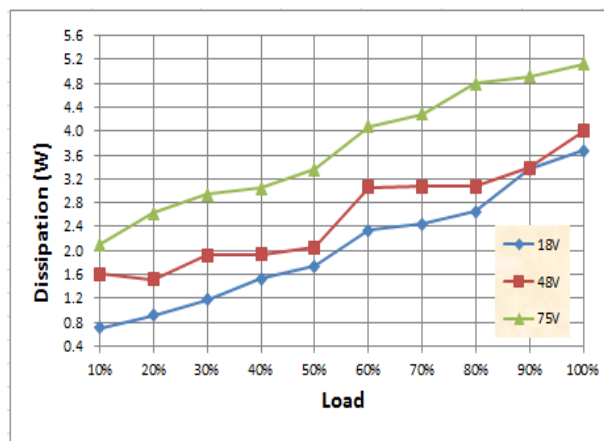
功率损失
