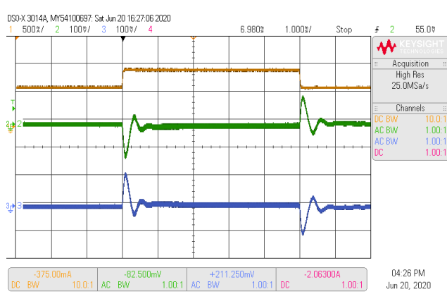
动态波形 (75%~50%~75% Iout)
