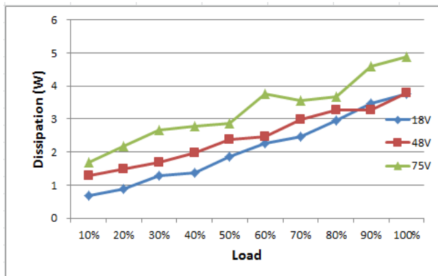
损耗曲线
