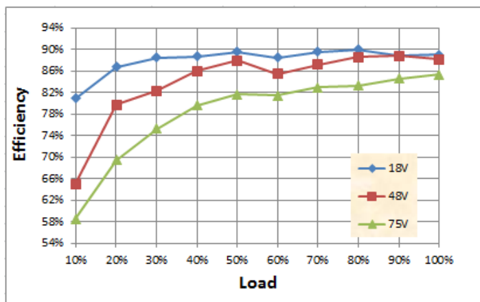
效率曲线
