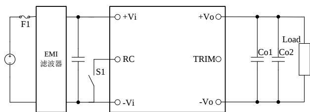
单路输出典型应用线路
