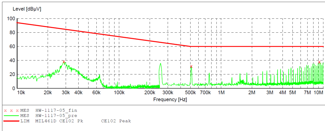
HQ200W-24S05B 模块传导测试结果（正线）
