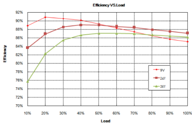
效率曲线
