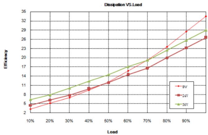
损耗曲线
