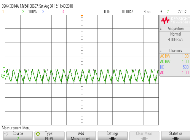
输出电压纹波波形(额定输入,满载)
