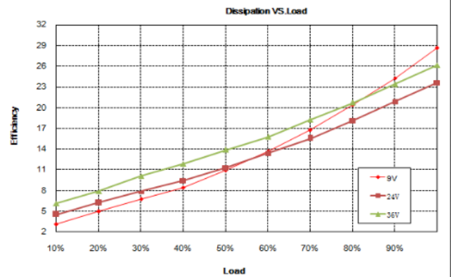
损耗曲线
