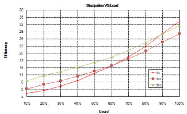
损耗曲线
