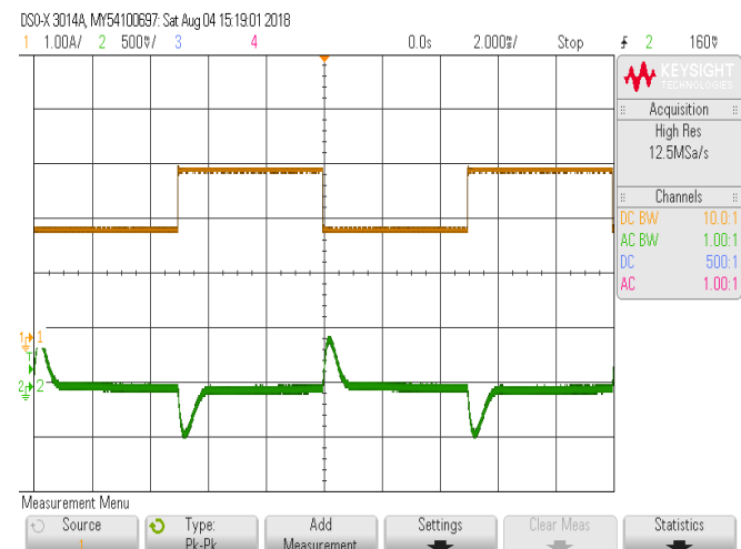
输出电压动态波形 (50%~75%~50% Iout)
