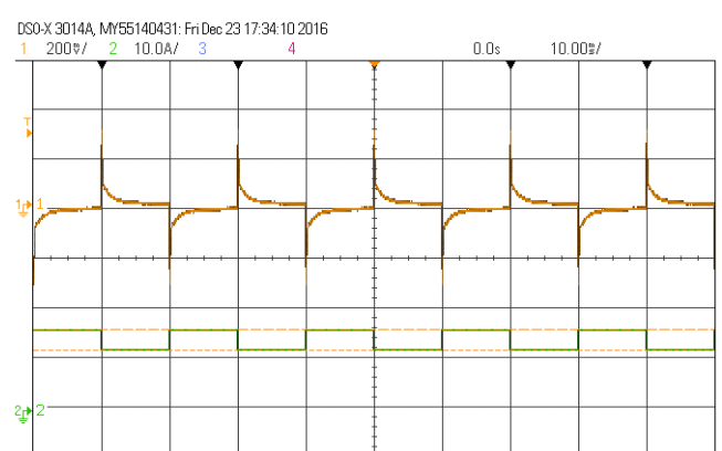
输出电压动态波形 (额定输入, 75%~100%~75% Iout)
