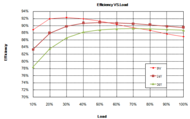
效率曲线
