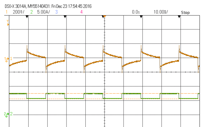
输出电压动态波形 (额定输入, 75%~100%~75% Iout)
