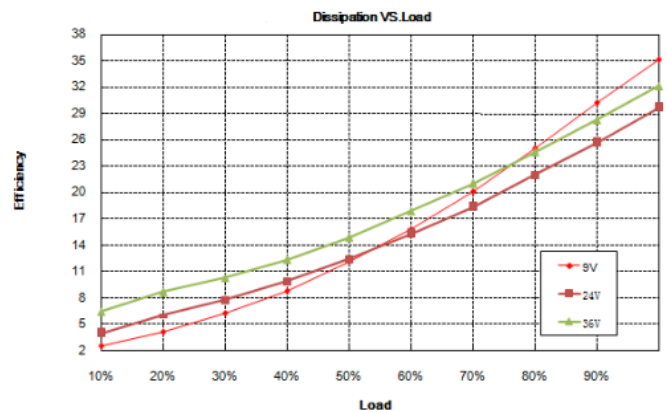
损耗曲线
