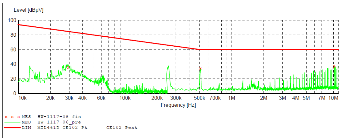
HQ200W-24S05B 模块传导测试结果（负线）
