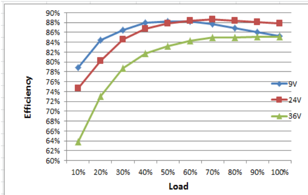
效率曲线
