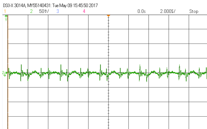
输出电压纹波波形(额定输入,满载)
