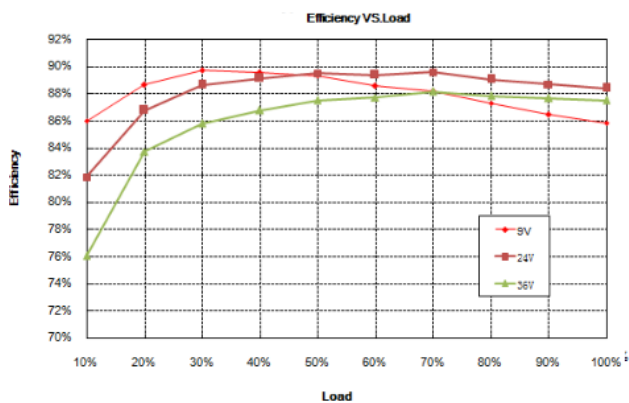
效率曲线
