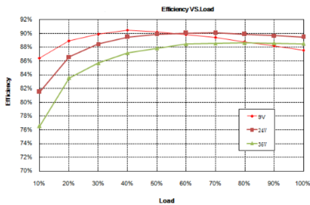
效率曲线
