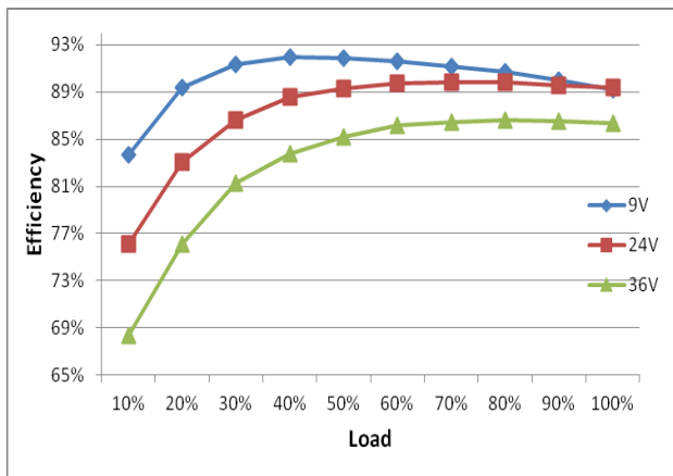
效率曲线
