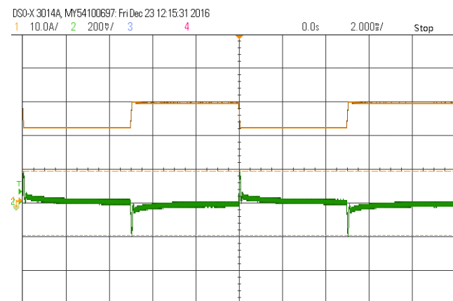
输出电压纹波波形 (75%~100%~75% Iout)
