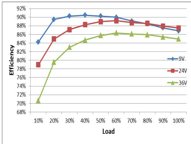
效率曲线
