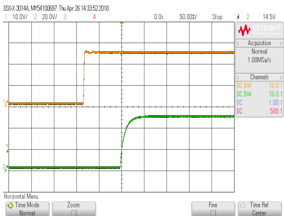
启动波形(额定输入,满载)
