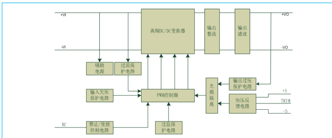
模块功能框图
