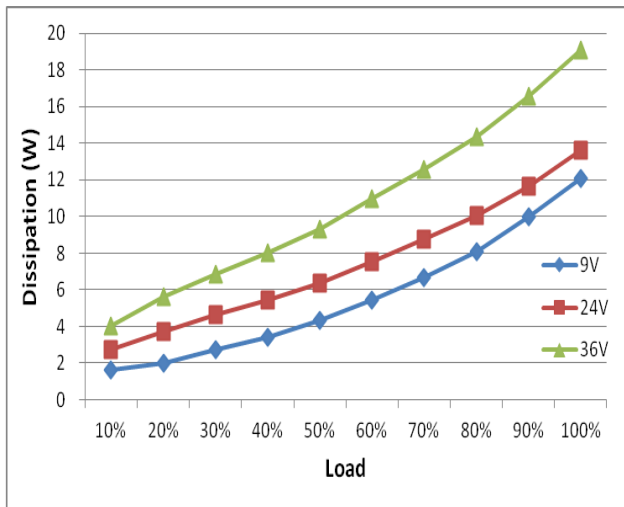
损耗曲线
