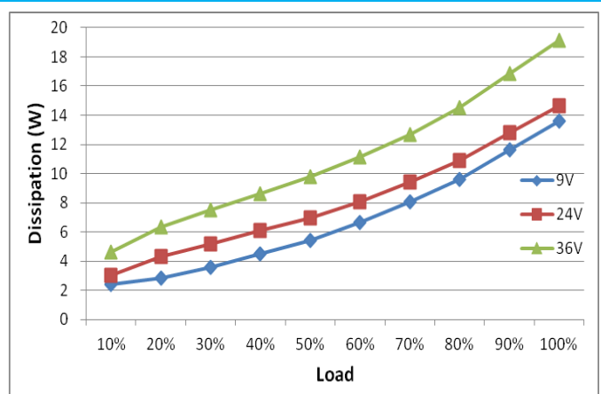
损耗曲线
