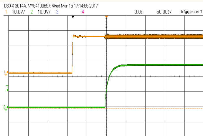
启动波形(额定输入,满载)
