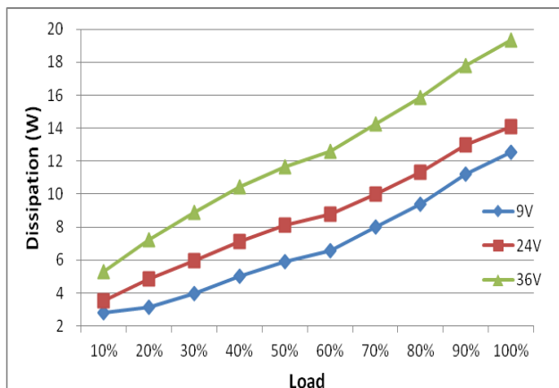
损耗曲线
