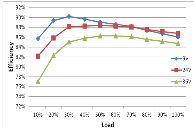
效率曲线
