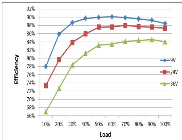
效率曲线
