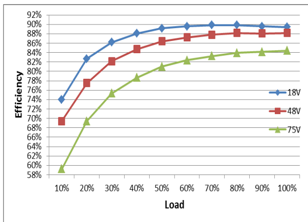
效率曲线
