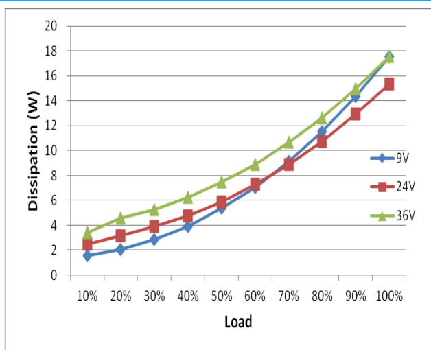
损耗曲线
