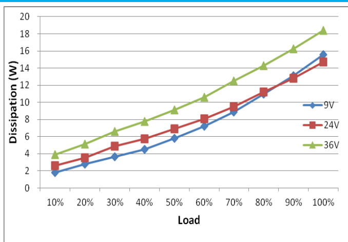
损耗曲线
