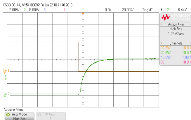
使能起机波形 (负逻辑)
