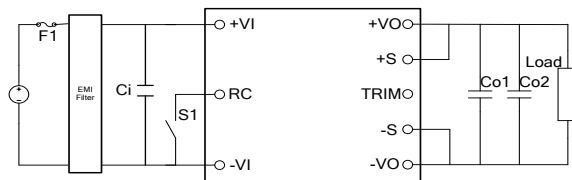
图 1 典型应用线路
