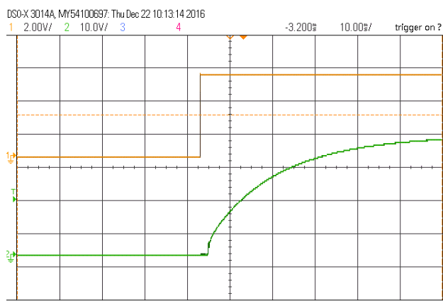
使能起机波形 (正逻辑)
