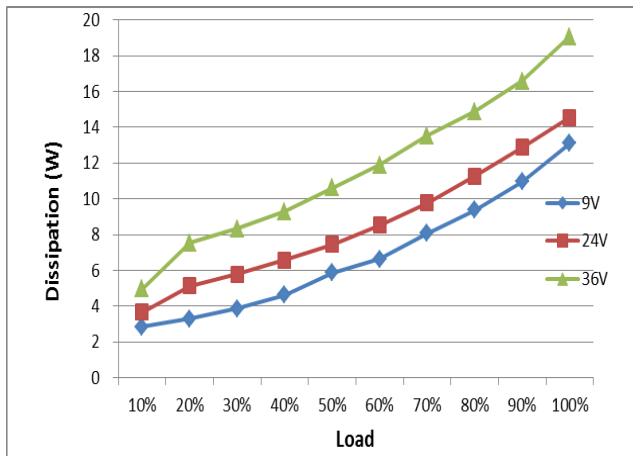
损耗曲线
