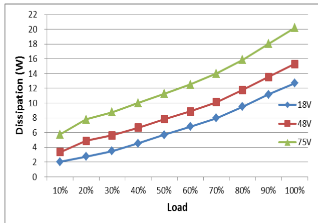
损耗曲线
