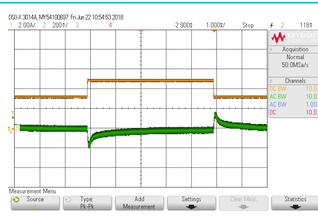
输出电压动态波形 (50%~75%~50% Iout)
