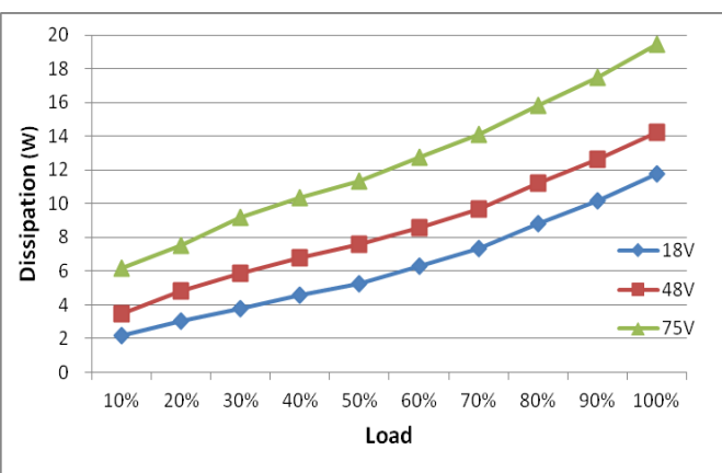
损耗曲线
