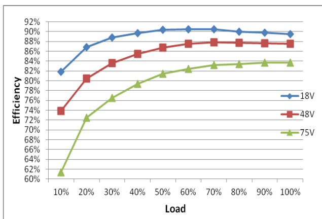
效率曲线
