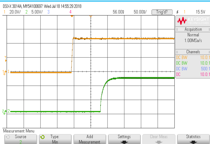
启动波形(额定输入,满载)
