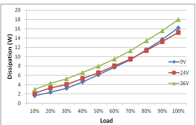
损耗曲线
