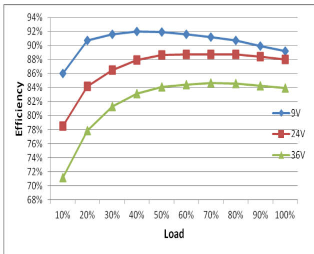
效率曲线
