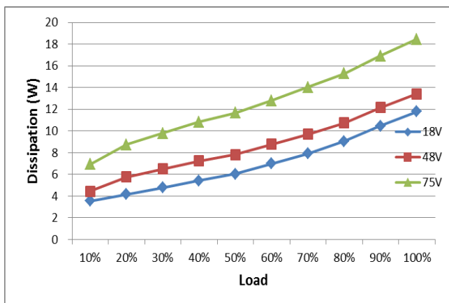
损耗曲线
