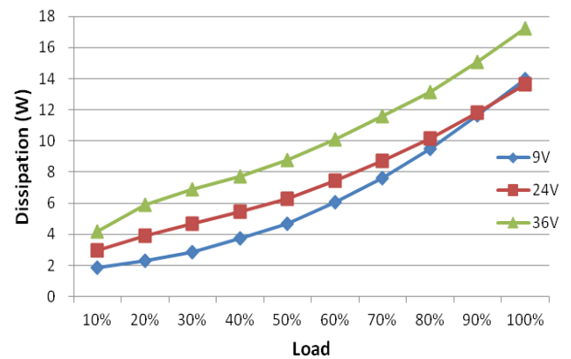
损耗曲线
