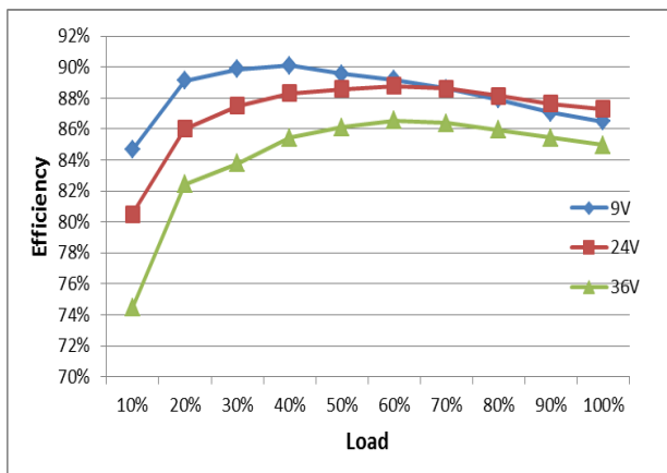
效率曲线
