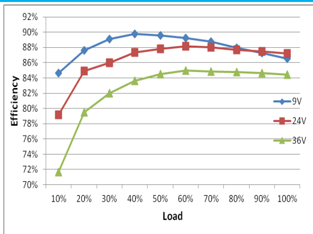
效率曲线
