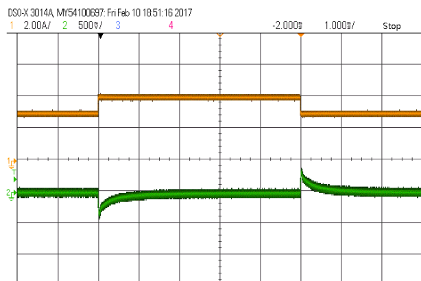
输出电压动态波形 (75%~100%~75% Iout)
