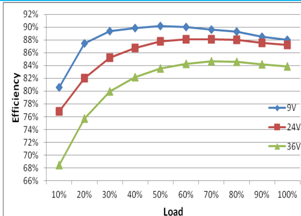
效率曲线
