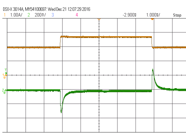
输出电压动态波形 (75%~100%~75% Iout)
