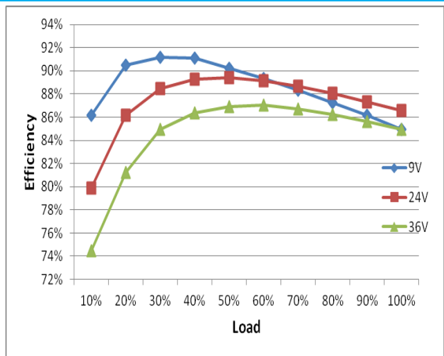
效率曲线
