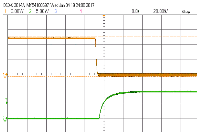
使能起机波形 (负逻辑) CH1: 使能引脚电压 CH2: 输出电压
