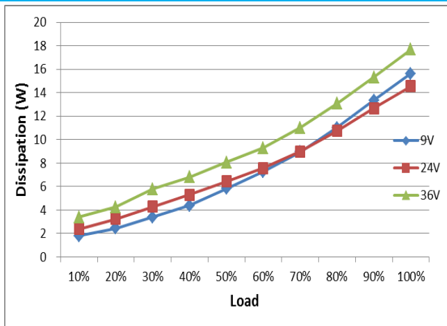
损耗曲线
