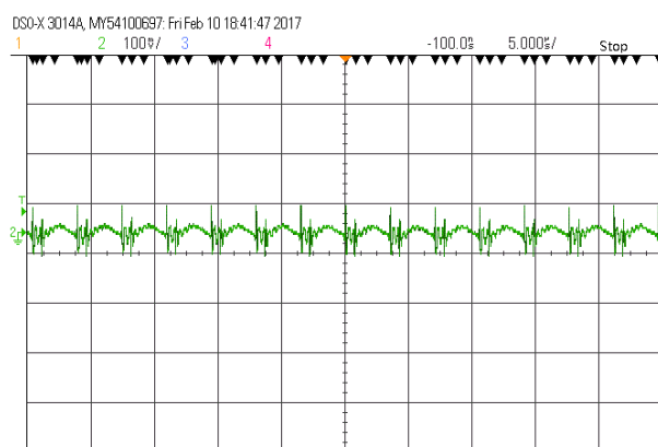
输出电压纹波波形(额定输入,满载)
