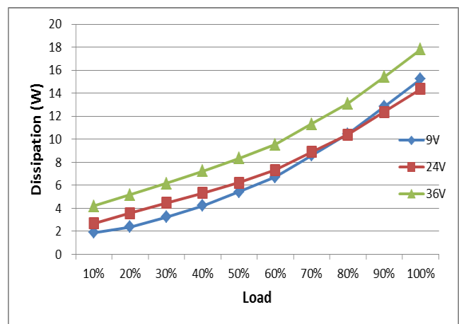
损耗曲线
