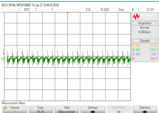
输出电压纹波波形(额定输入,满载)
