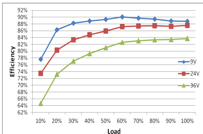
效率曲线
