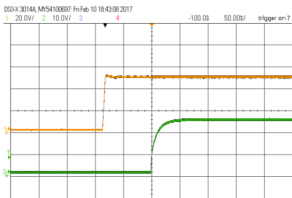
启动波形(额定输入,满载)
