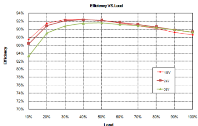
效率曲线
