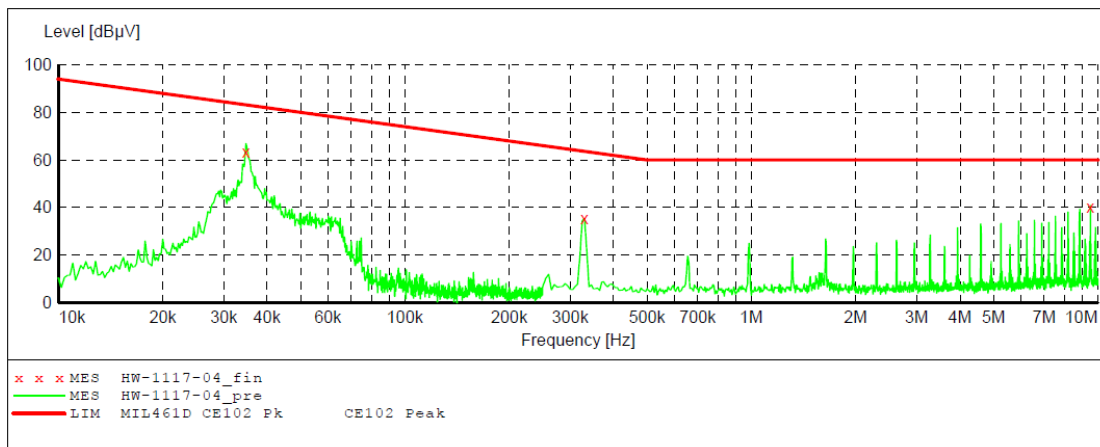
HQ350-24S28B 模块传导测试结果（正线）
