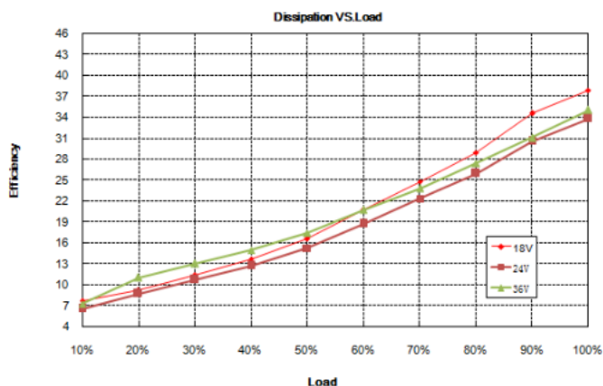
损耗曲线
