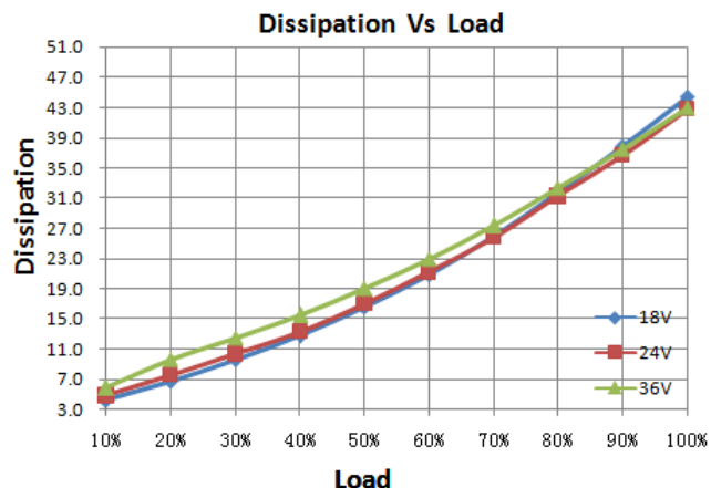
损耗曲线
