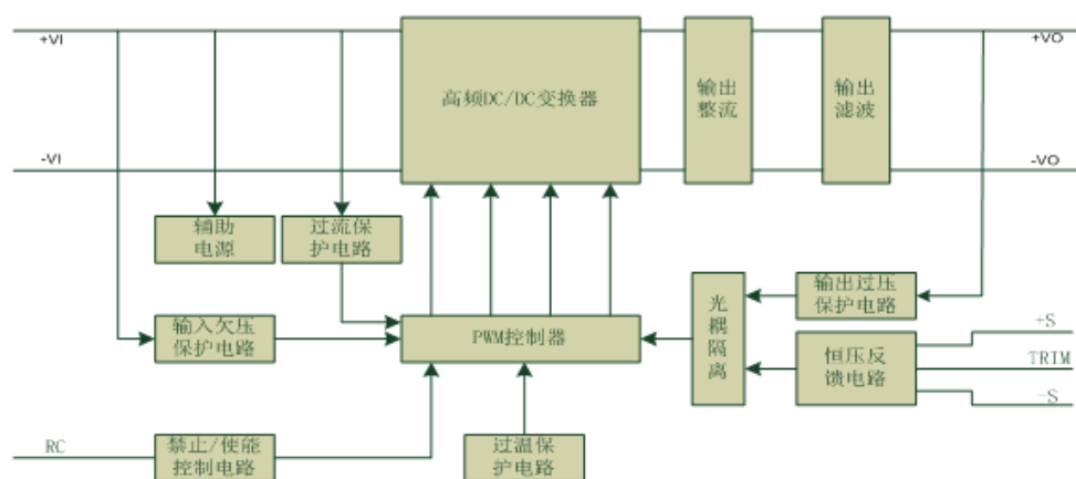
模块功能框图
