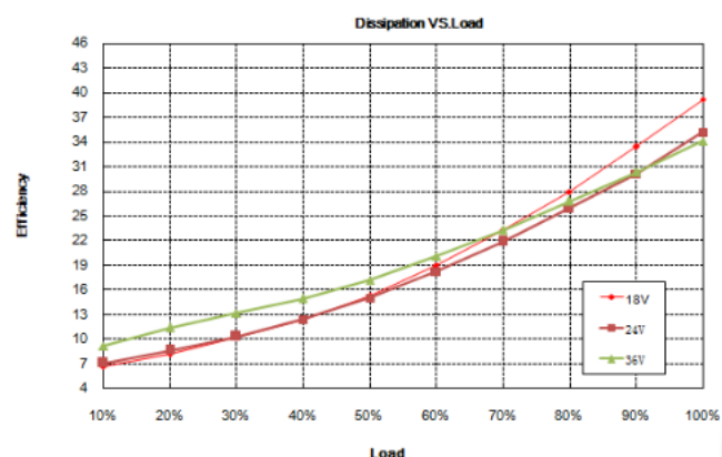
损耗曲线
