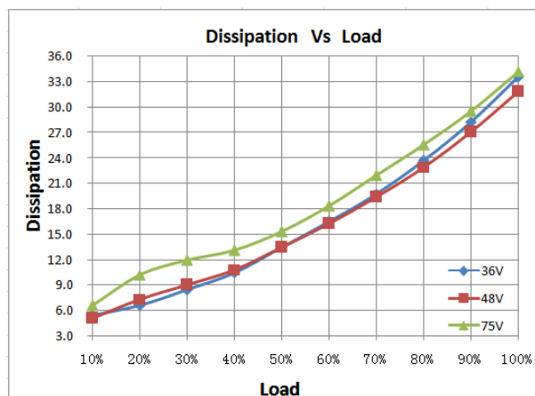
损耗曲线
