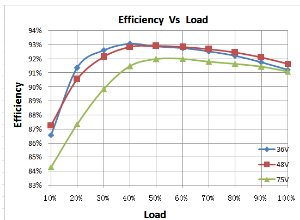
效率曲线
