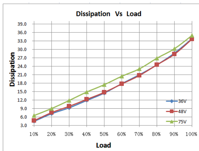
损耗曲线
