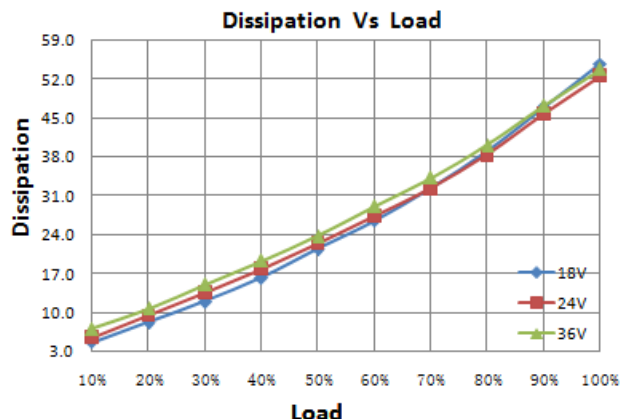
损耗曲线
