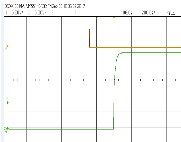
使能起机波形 (负逻辑) CH1: 使能引脚电压 CH2: 输出电压
