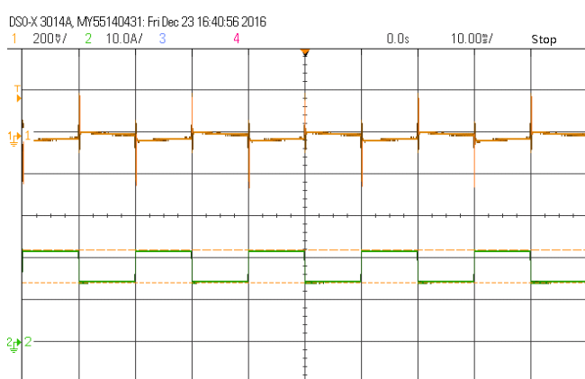
输出电压动态波形 (额定输入, 50%~75%~50% Iout)
