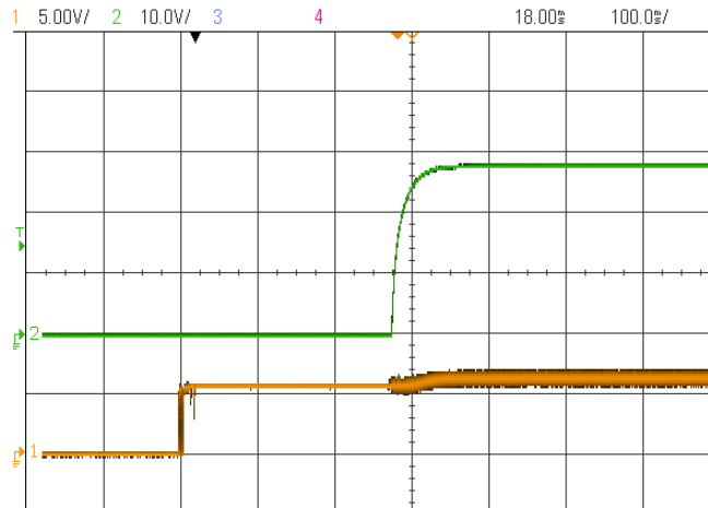
使能起机波形 (正逻辑) CH1: 使能引脚电压 CH2: 输出电压
