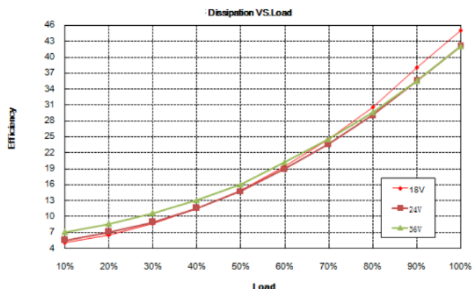
损耗曲线
