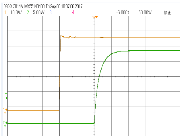
启动波形(额定 48V 输入,满载) CH1:输入电压 CH2:输出电压
