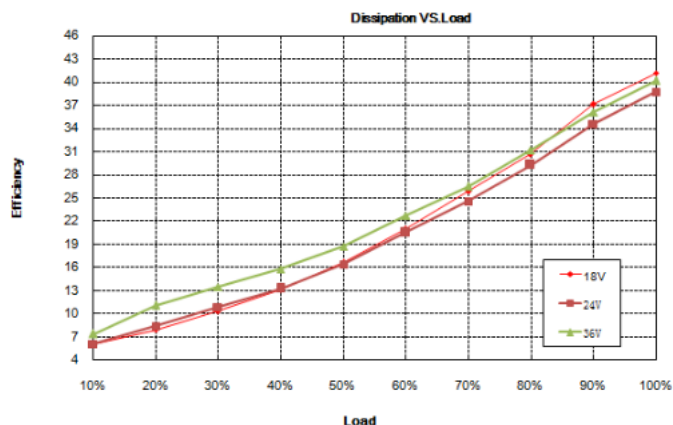
损耗曲线
