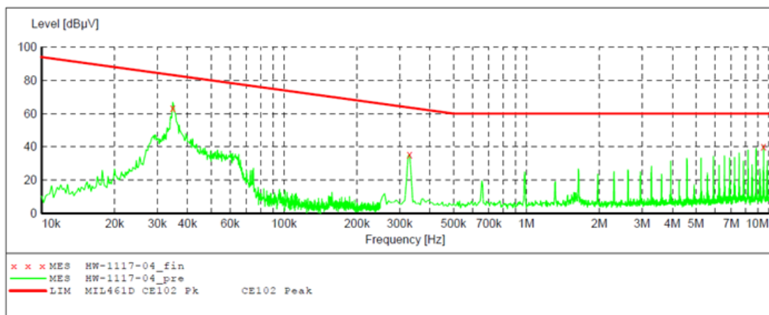
HQ350-24S28B 模块传导测试结果（负线）
