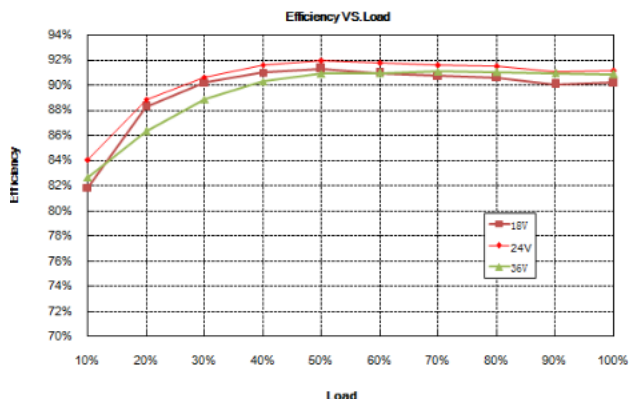
效率曲线
