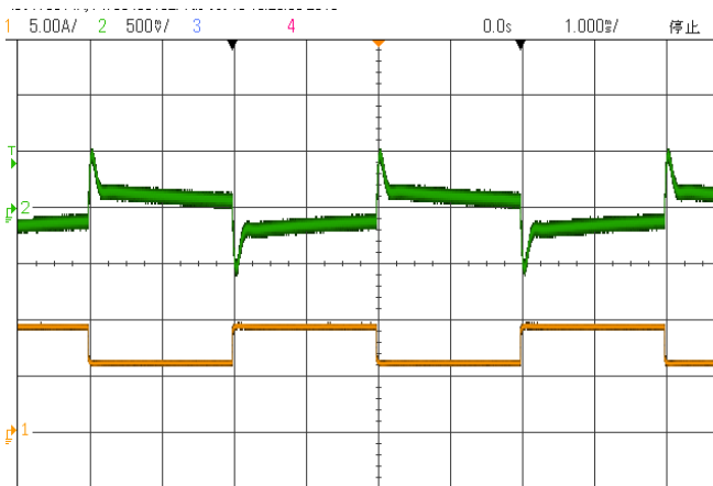
动态波形 (50%~75%~50% Iout)
