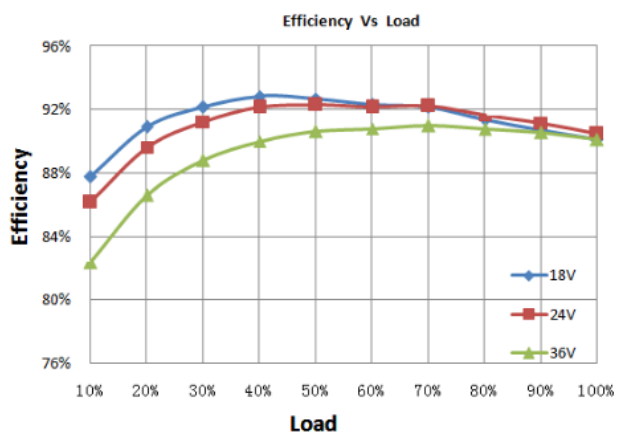
效率曲线
