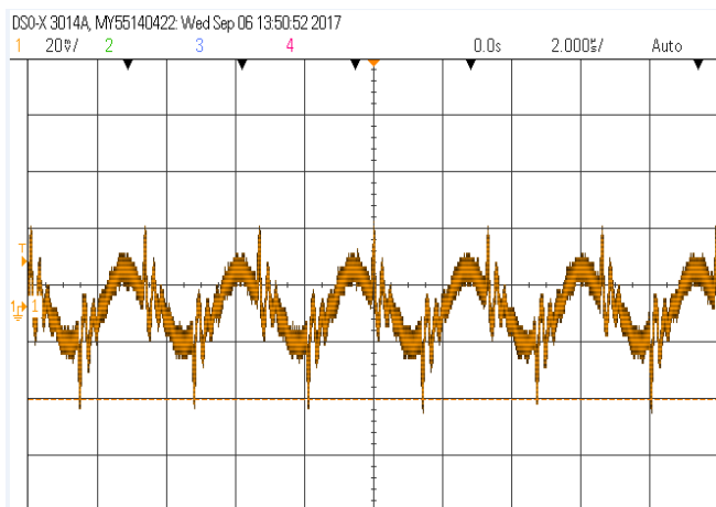
输出电压纹波波形(额定 48V 输入,满载)
