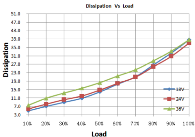
损耗曲线
