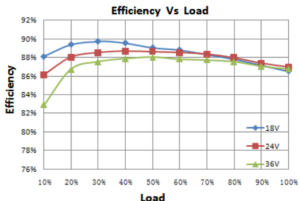
效率曲线
