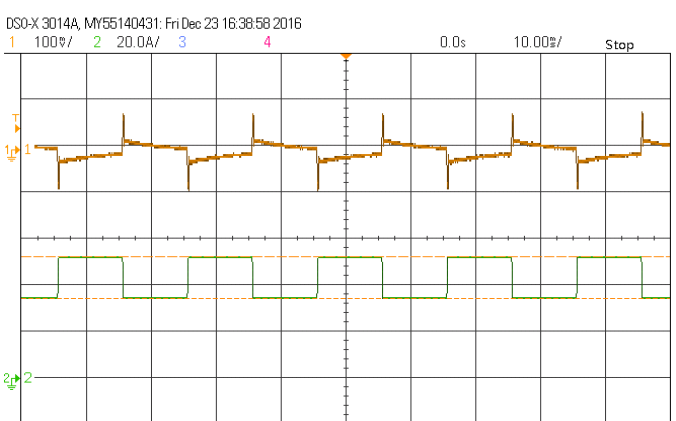
输出电压动态波形 (额定输入, 50%~75%~50% Iout)
