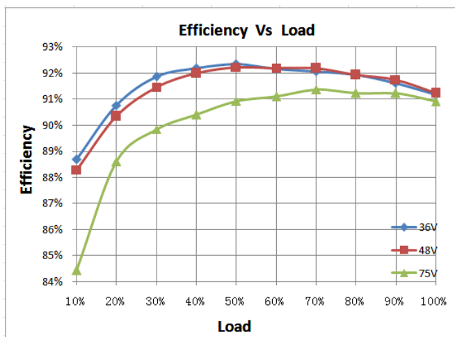
效率曲线
