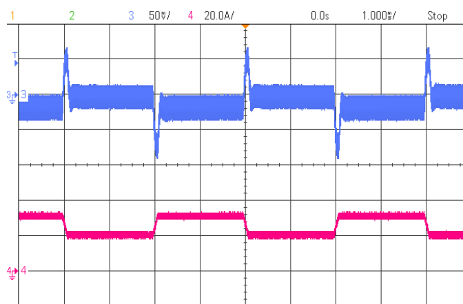
输出电压动态波形 (额定输入, 50%~75%~50% Iout)
