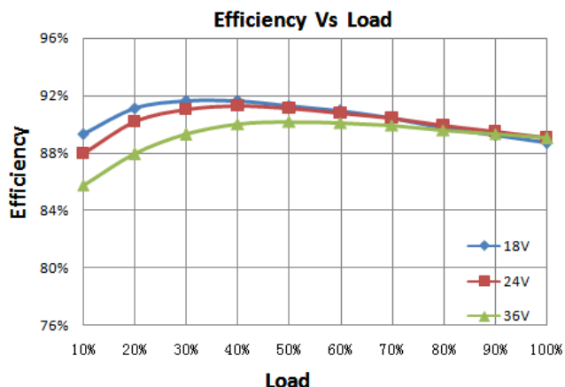
效率曲线
