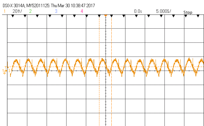
纹波(额定 300VDC 输入,满载)
