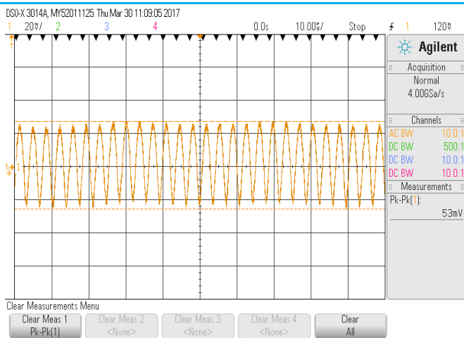
纹波(额定 300VDC 输入,满载)
