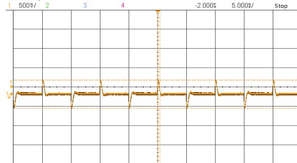
动态波形 (75%~100%~75% Iout)
