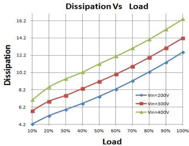
损耗曲线
