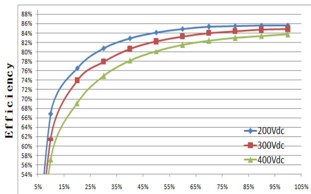
效率曲线
