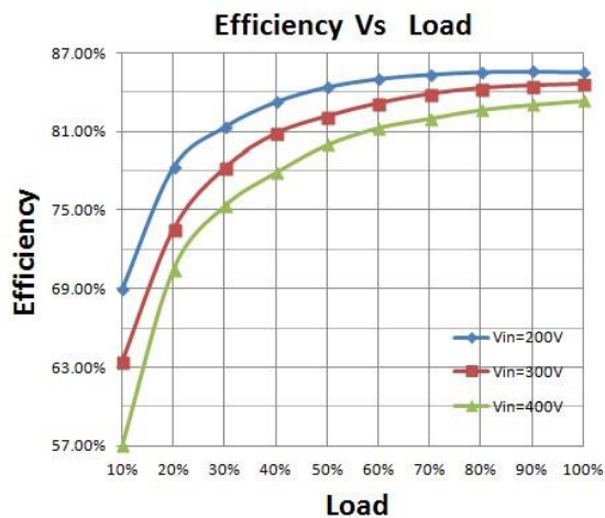
效率曲线
