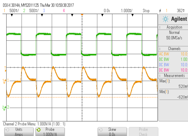
动态波形 (75%~100%~75% Iout)
