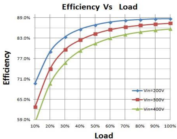
效率曲线
