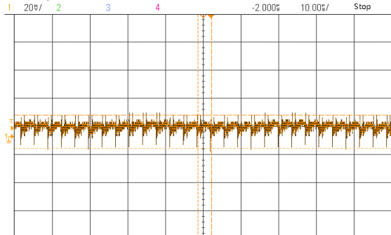
纹波(额定 300VDC 输入,满载)
