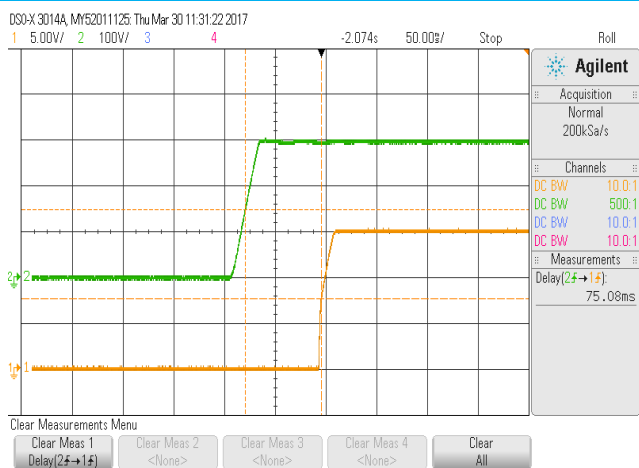
启动波形(额定 300VDC 输入,满载) CH1:输入电压 CH2:输出电压
