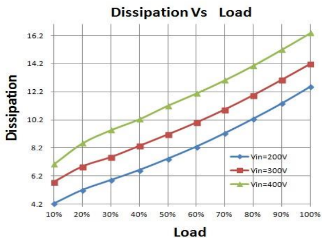
损耗曲线
