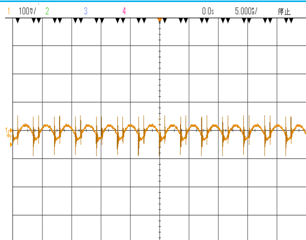
纹波(额定 300VDC 输入,满载)
