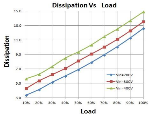
损耗曲线
