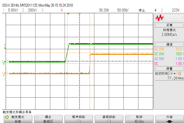
启动波形(额定 300VDC 输入,满载) CH1:输出电压 CH2:输入电压
