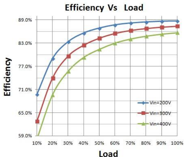
效率曲线
