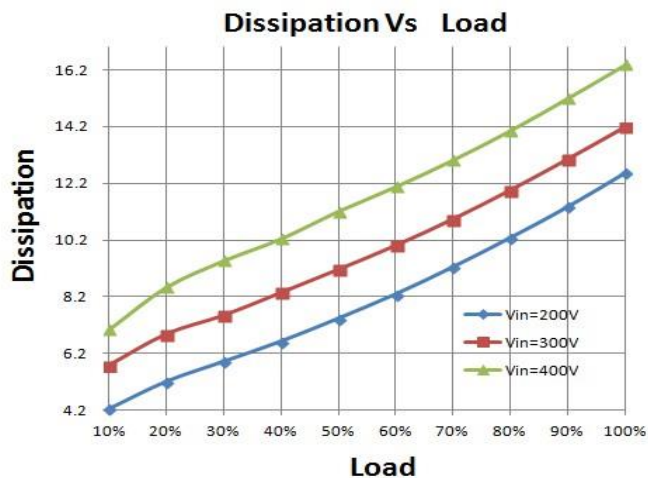
损耗曲线
