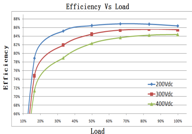
效率曲线
