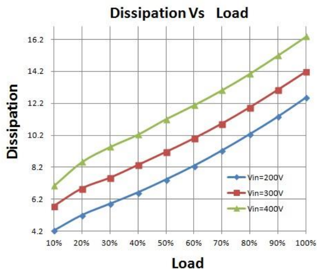
损耗曲线
