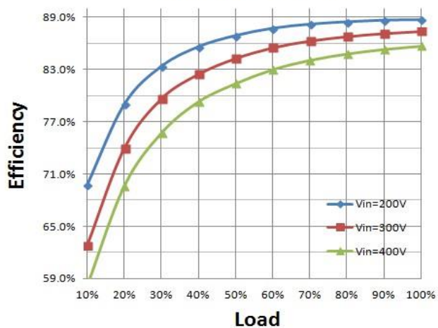
效率曲线
