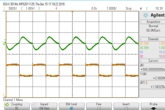
动态波形 (75%~100%~75% Iout)
