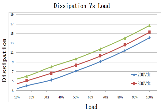
损耗曲线
