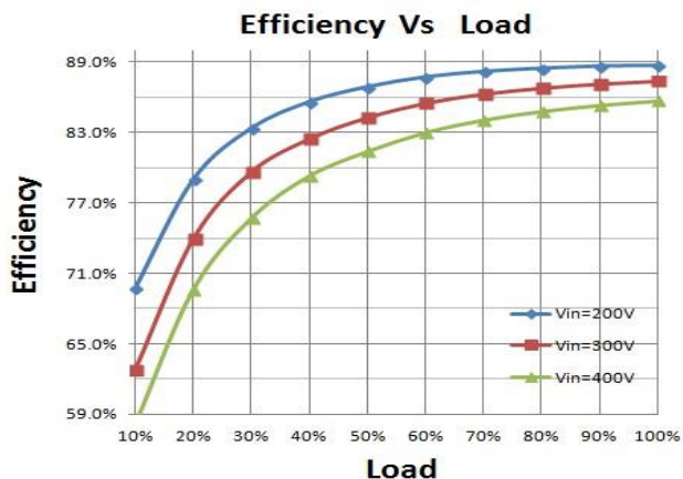
效率曲线
