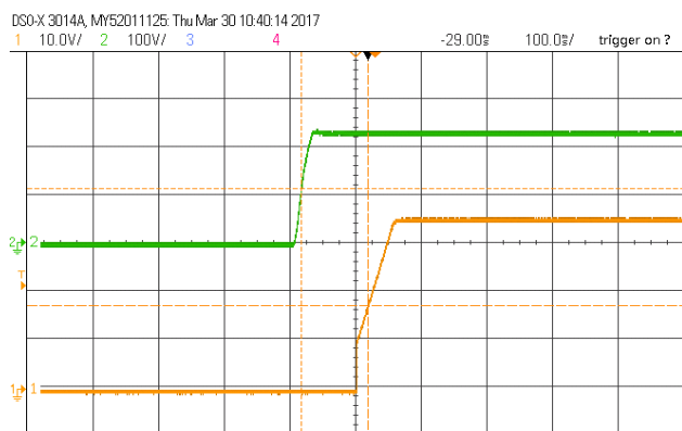
启动波形(额定 300VDC 输入,满载) CH1:输入电压 CH2:输出电压
