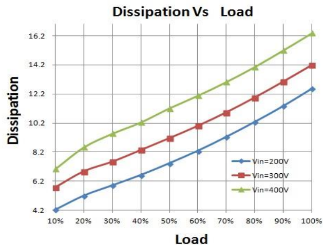
损耗曲线
