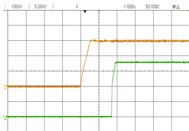
启动波形(额定 300VDC 输入,满载) CH1:输入电压 CH2:输出电压
