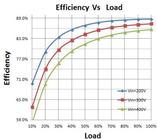
效率曲线
