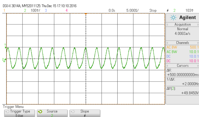
纹波(额定 300VDC 输入,满载)
