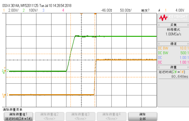
启动波形(额定 300VDC 输入,满载) CH1:输出电压 CH2:输入电压
