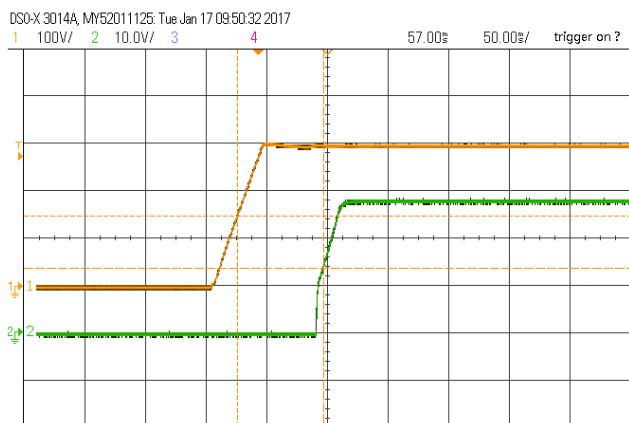
启动波形(额定 300VDC 输入,满载) CH1:输入电压 CH2:输出电压
