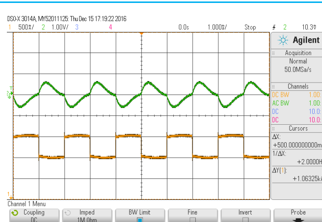
动态波形 (75%~100%~75% Iout)
