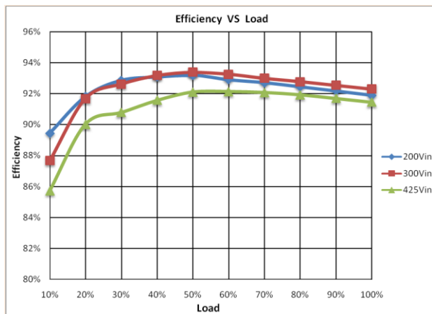
效率曲线
