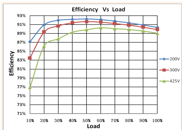
效率曲线
