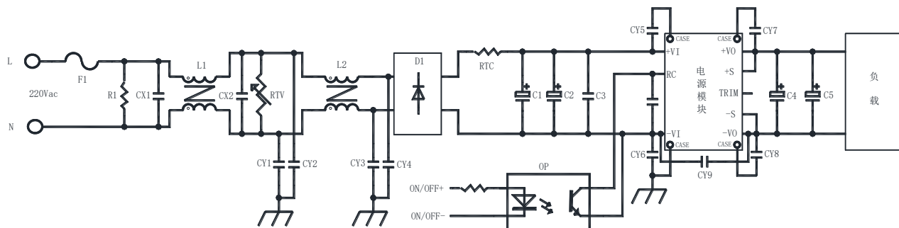
图 1 典型应用线路图
