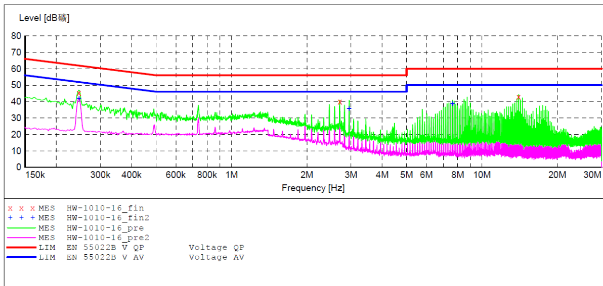
图 2 HQ500-300S28B 模块传导测试结果
