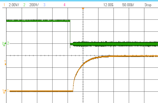
使能起机波形 (负逻辑) CH1: 输出电压 CH2: 使能引脚电压
