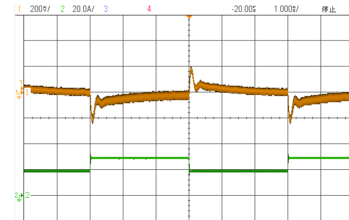
输出电压动态波形 (额定输入, 75%~50%~75% Io)
