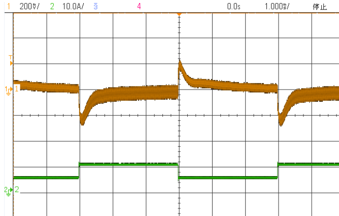
输出电压动态波形 (额定输入, 25%~50%~25% Io)
