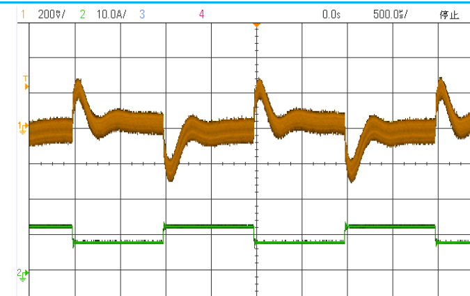
输出电压动态波形(额定输入, 75%~50%~75% Io)
