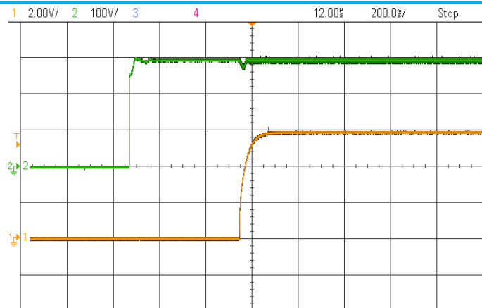
启动波形(额定输入, 满载) CH1:输出电压 CH2:输入电压
