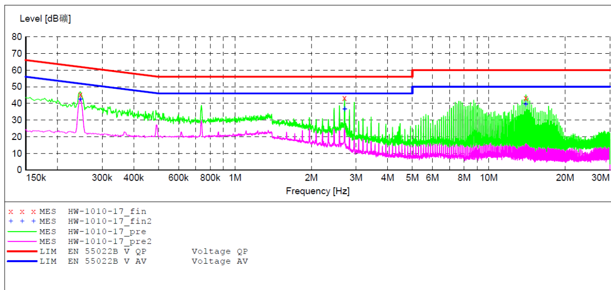
图 3 HQ500-300S28B 模块传导测试结果
