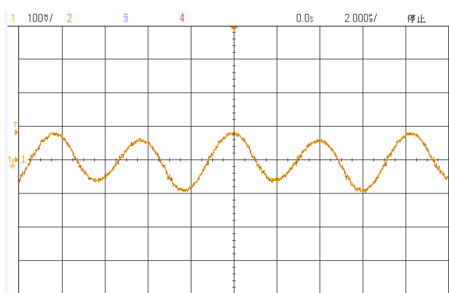
输出纹波电压波形(额定输入, 满载)
