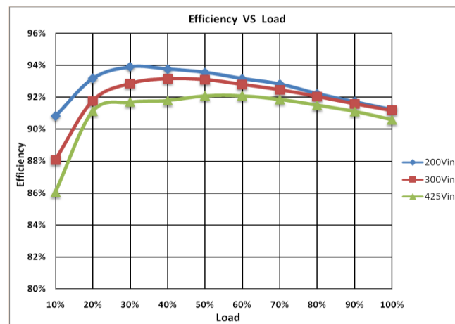
效率曲线
