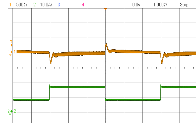
输出电压动态波形 (额定输入, 25%~50%~25% Io)
