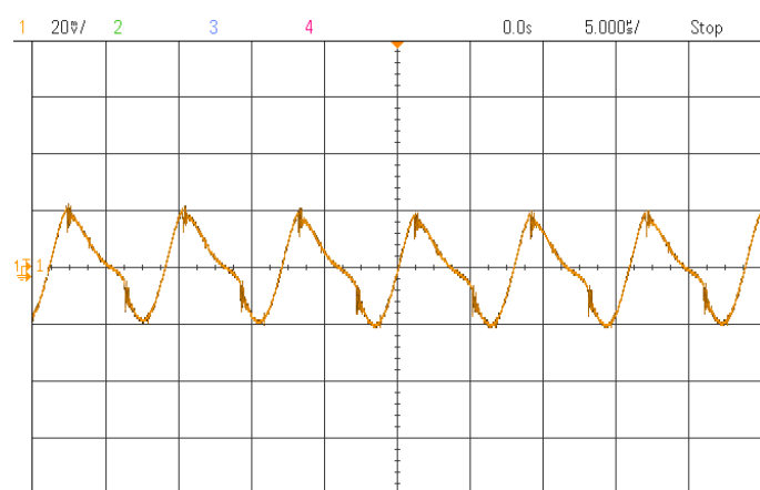
输出电压纹波波形(额定输入,满载)
