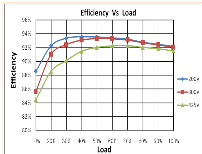
效率曲线
