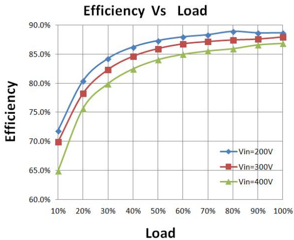
效率曲线
