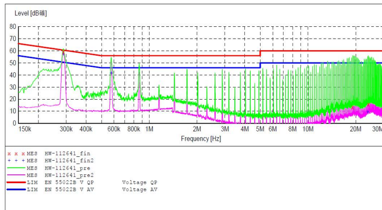
HQ250-300S15B 模块传导测试结果
