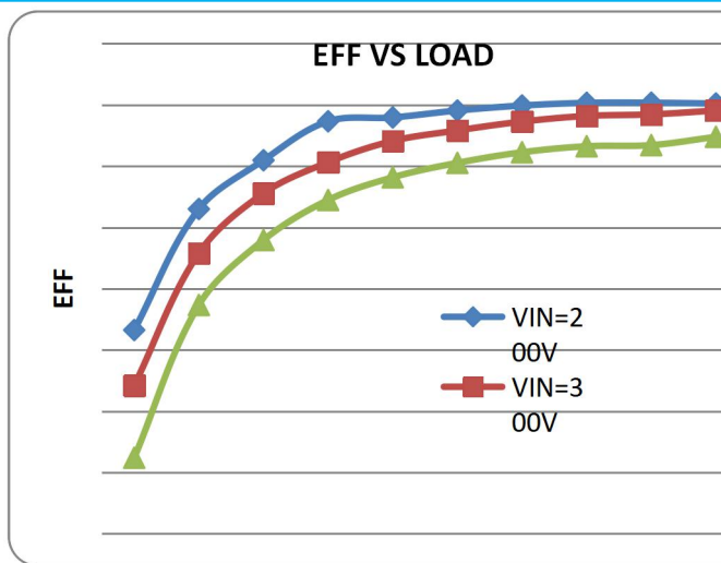
效率曲线
