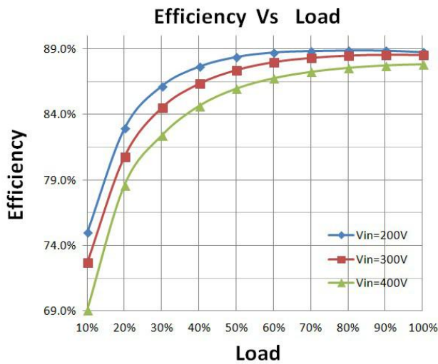
效率曲线
