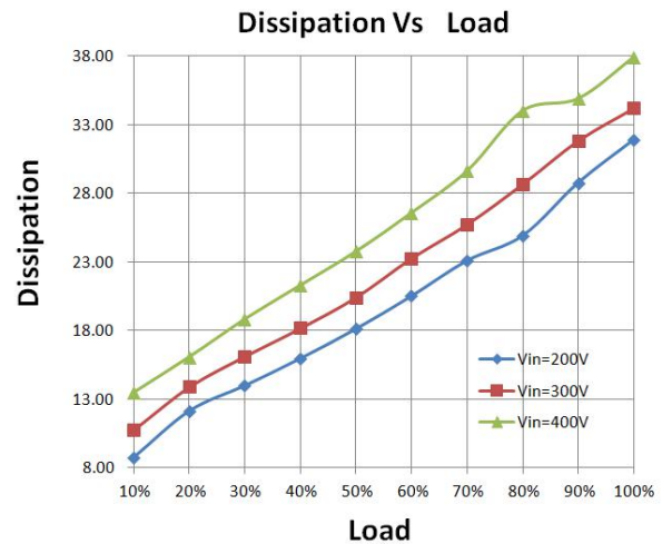
损耗曲线
