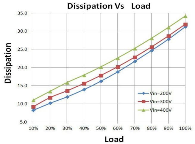
损耗曲线
