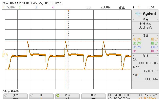
动态波形 (75%~100%~75% Iout)
