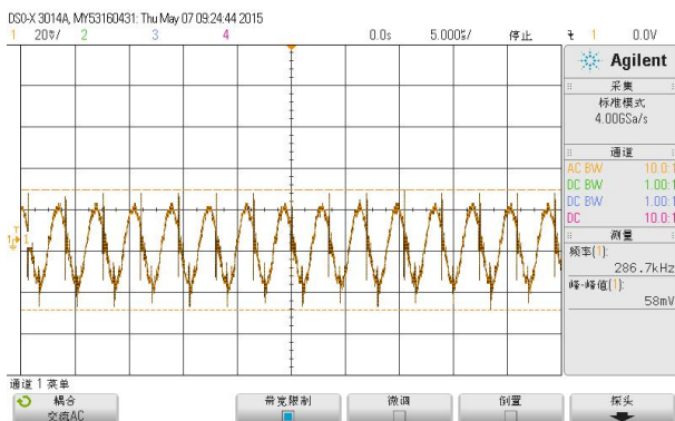
纹波(额定 300VDC 输入,满载)
