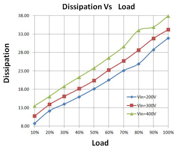
损耗曲线
