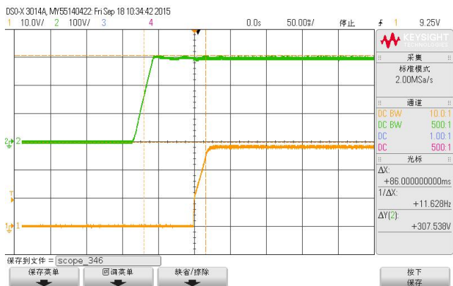
启动波形(额定 300VDC 输入,满载)
