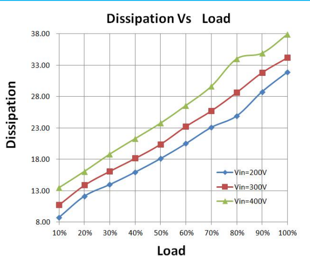
损耗曲线
