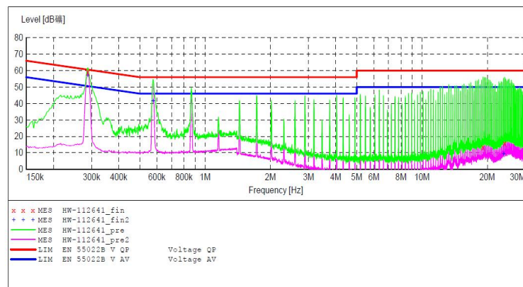
HQ250-300S28B 模块传导测试结果
