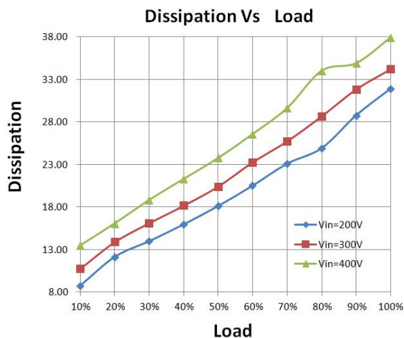
损耗曲线
