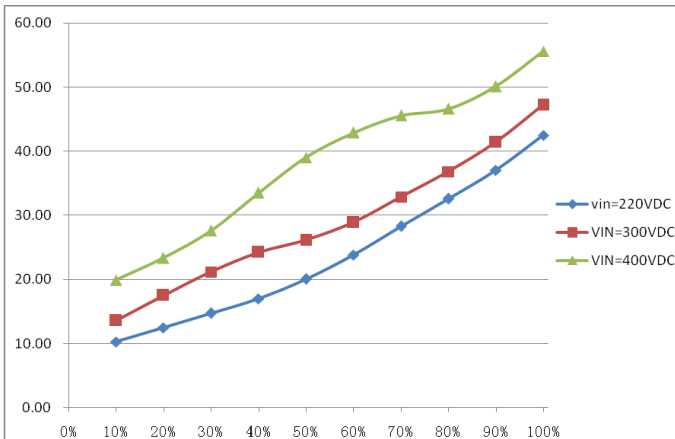
损耗曲线
