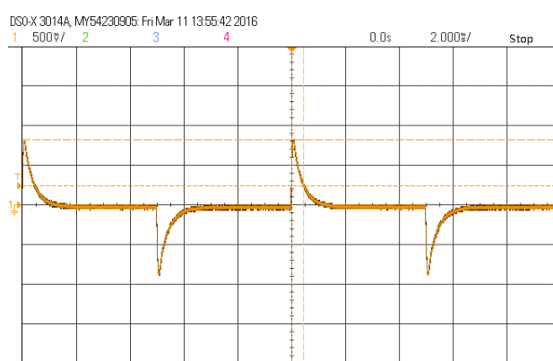
动态波形 (50%~75%~50%Iout)
