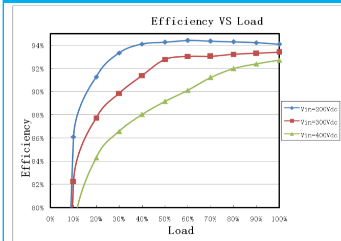
效率曲线
