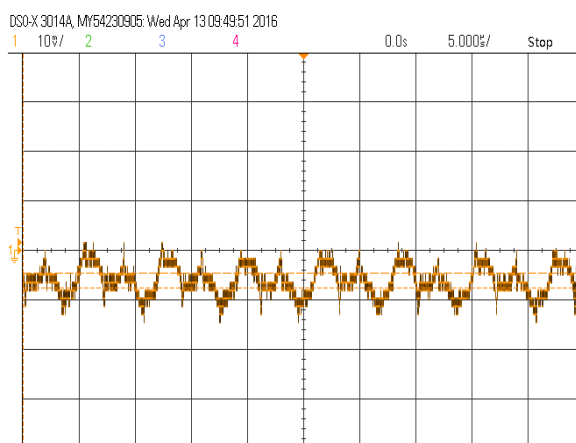
纹波(额定 300VDC 输入,满载)
