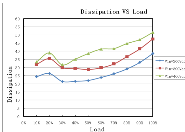
损耗曲线
