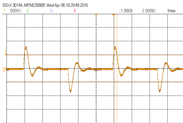
动态波形 (50%~75%~50%Iout)
