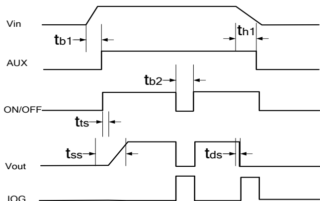
FQ600-300SXXB 正逻辑模块电源时序图
