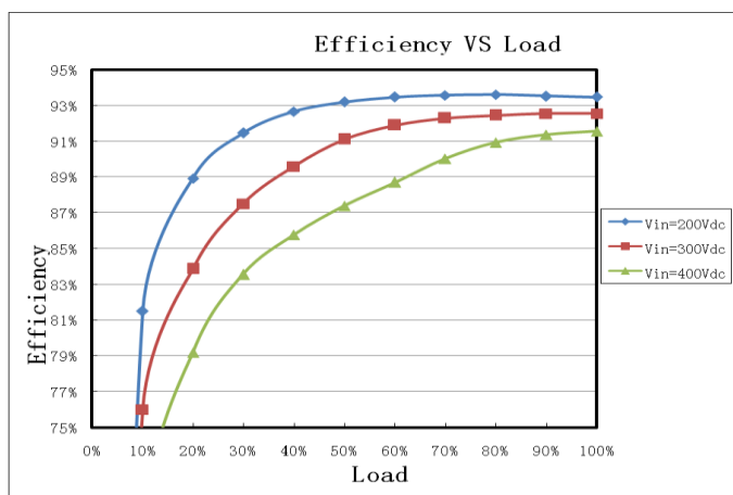
效率曲线
