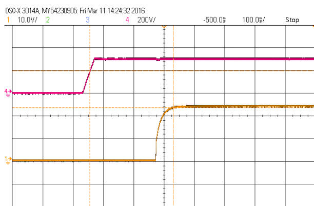
启动波形(额定 300VDC 输入,满载) CH4:输入电压 CH1: 输出电压
