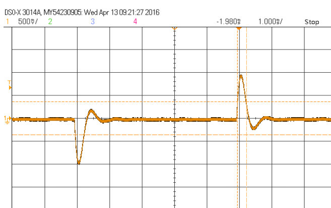
动态波形 (50%~75%~50%Iout)
