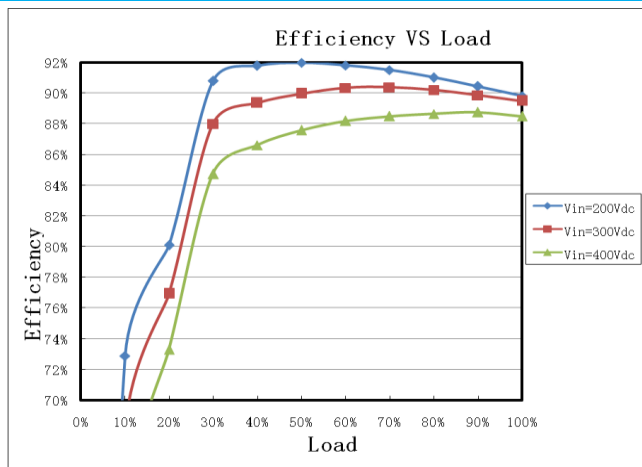
效率曲线
