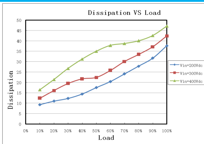
损耗曲线
