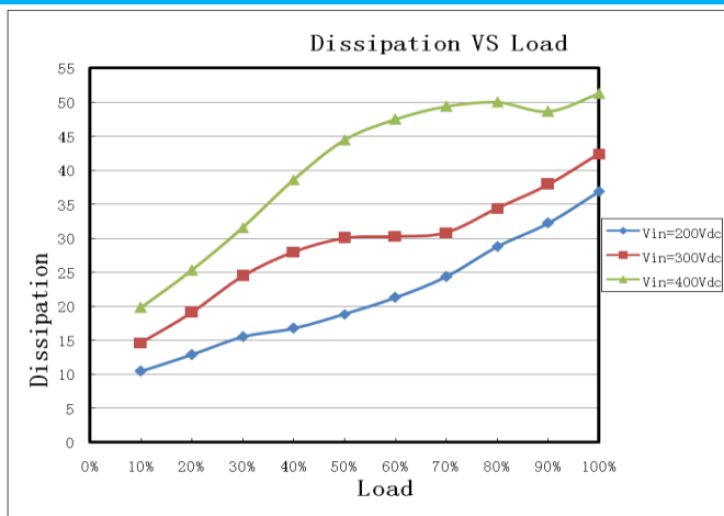
损耗曲线
