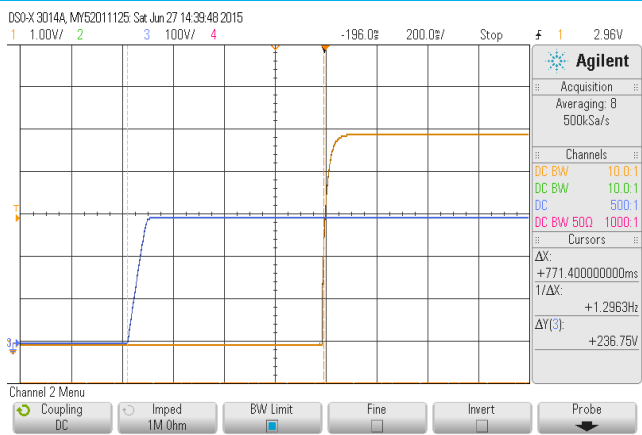
启动波形(额定 300VDC 输入,满载) CH1:输出电压 CH3:输入电压
