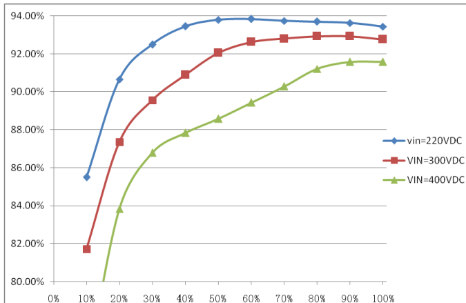
效率曲线
