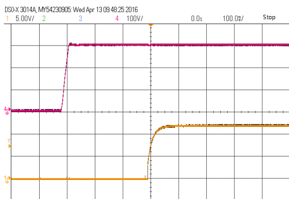
启动波形(额定 300VDC 输入,满载) CH4:输入电压 CH1: 输出电压
