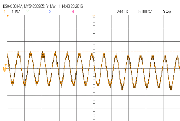
纹波(额定 300VDC 输入,满载)
