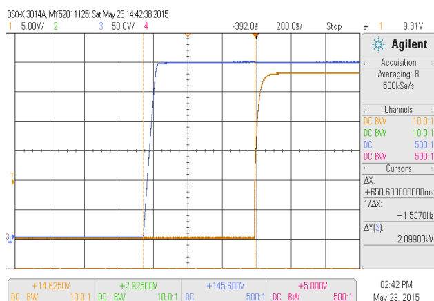
启动波形(额定 300VDC 输入,满载) CH3: 输入电压 CH1 输出电压
