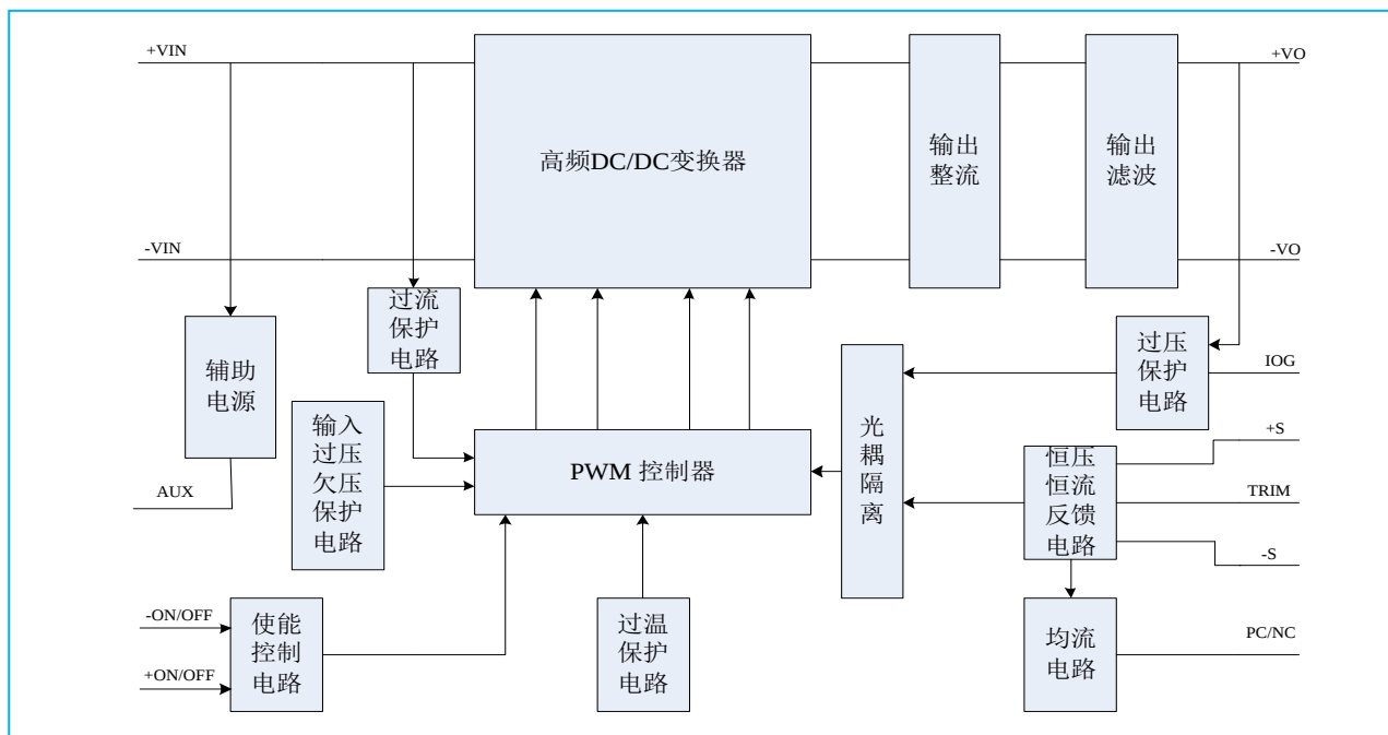
模块功能框图
