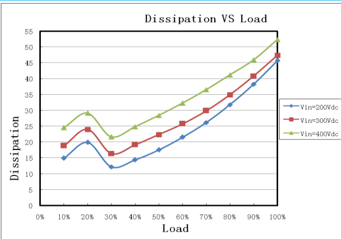
损耗曲线
