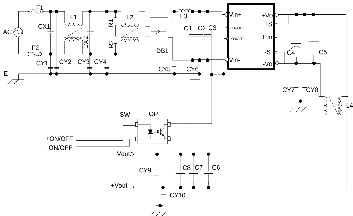
典型应用线路
