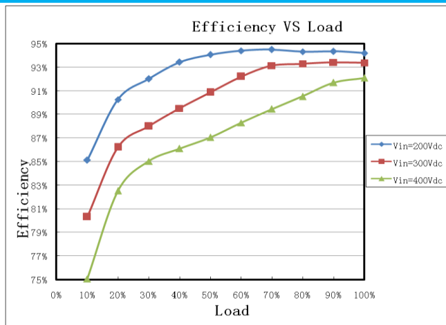
效率曲线
