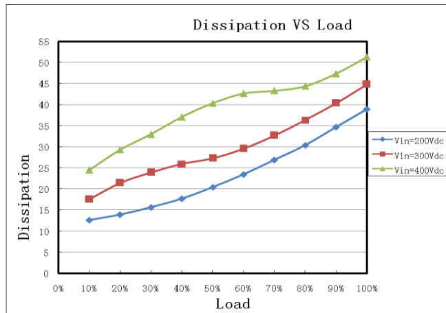
损耗曲线
