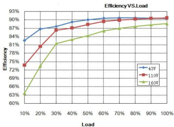
效率曲线
