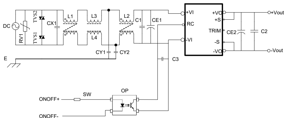
HQ200W-110S05B /12B/18B/24B EMI 滤波器参数如下:
