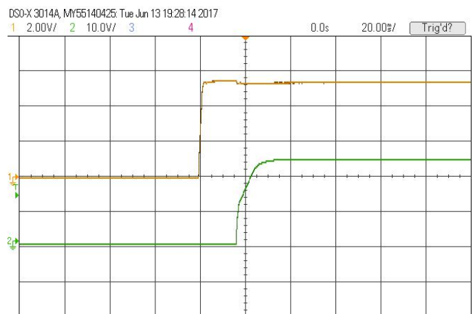
使能起机波形 (正逻辑)
