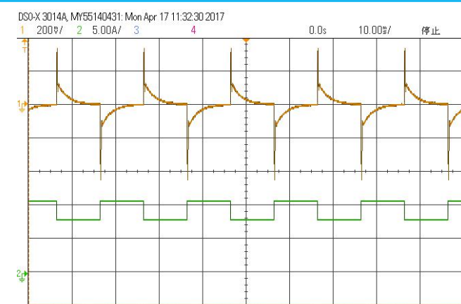
输出电压动态波形 (额定输出, 75%~100%~75% Iout)
