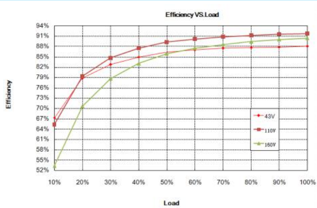
效率曲线
