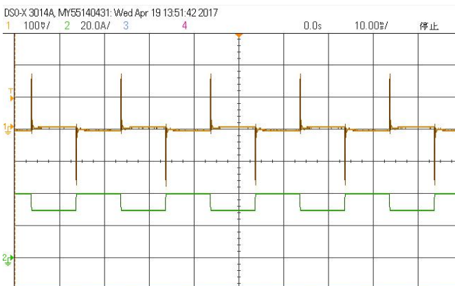
输出电压动态波形 (额定输出, 75%~100%~75% Iout)
