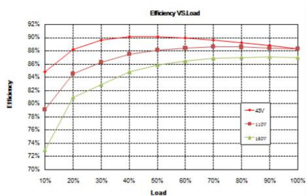
效率曲线
