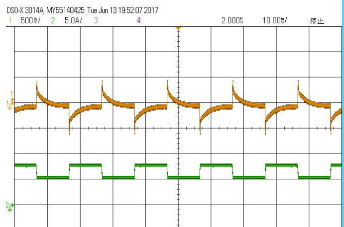
输出电压动态波形 (额定输出, 75%~100%~75% Iout)
