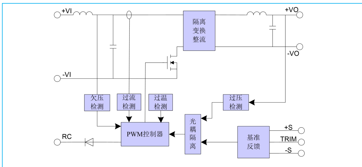
模块功能框图
