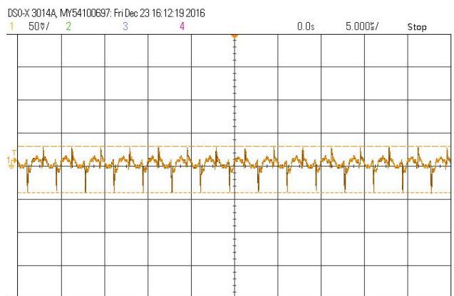
输出电压纹波(额定输入, 满载)
