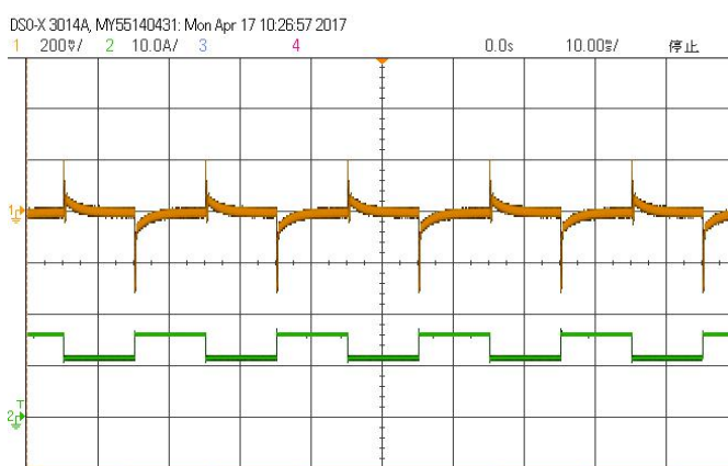
输出电压动态波形 (额定输出, 75%~100%~75% Iout)
