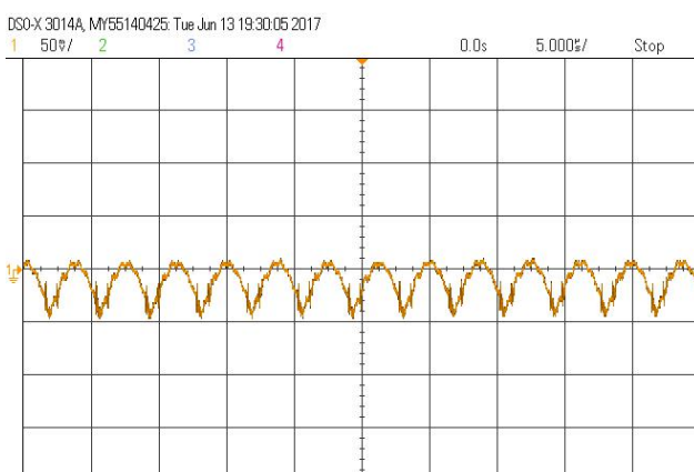
输出电压纹波(额定输入, 满载)
