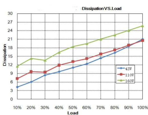
损耗曲线
