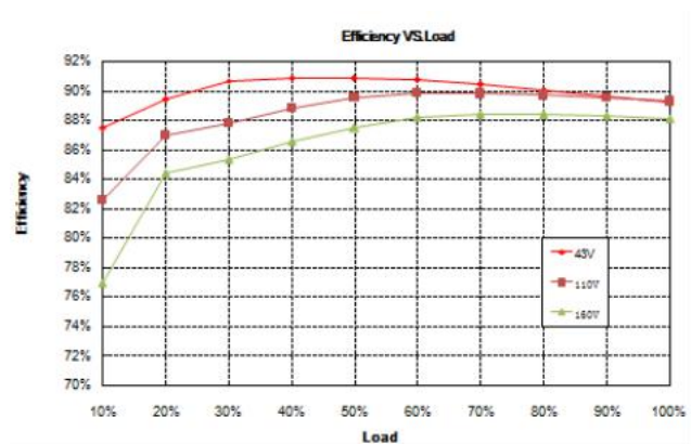
效率曲线
