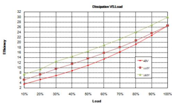
损耗曲线
