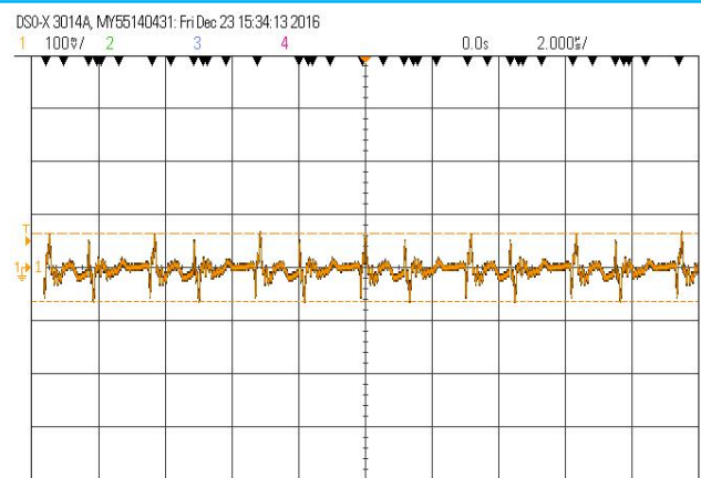
输出电压纹波(额定输入, 满载)
