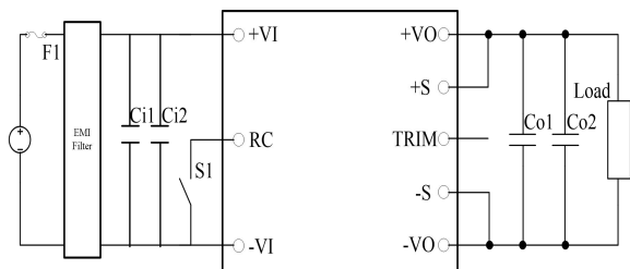
图 1 典型应用线路
