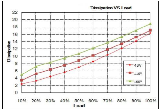
损耗曲线
