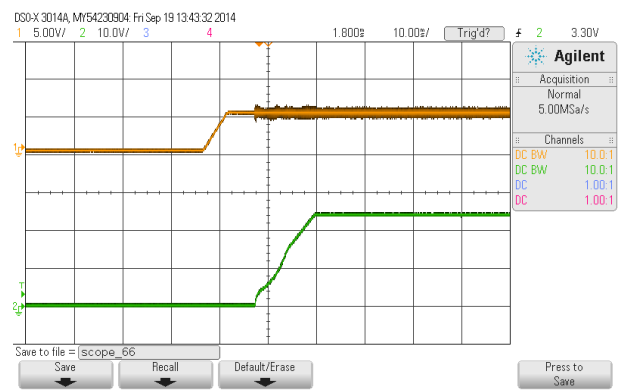
使能起机波形 (正逻辑)
