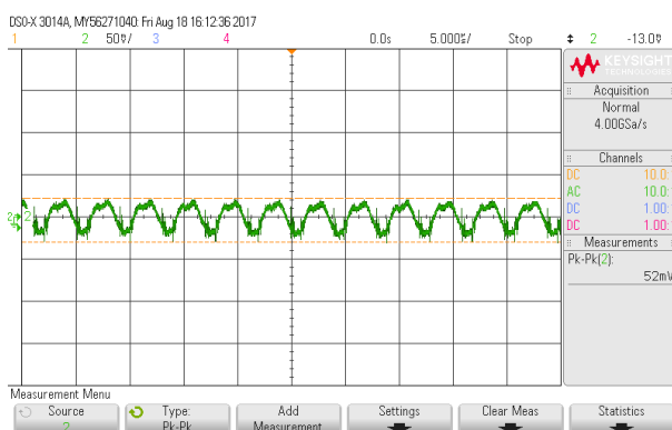
输出电压纹波(额定输入, 满载)
