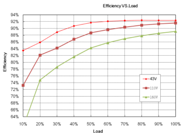
效率曲线
