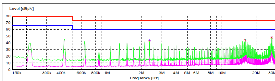
EQ100W-110S24B 模块传导测试结果
