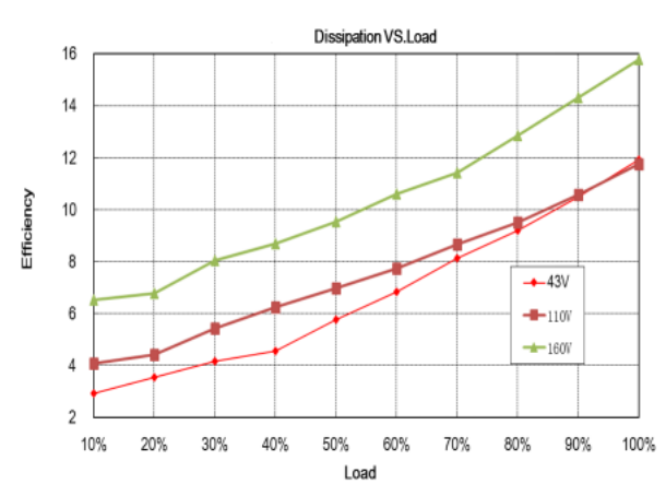
损耗曲线
