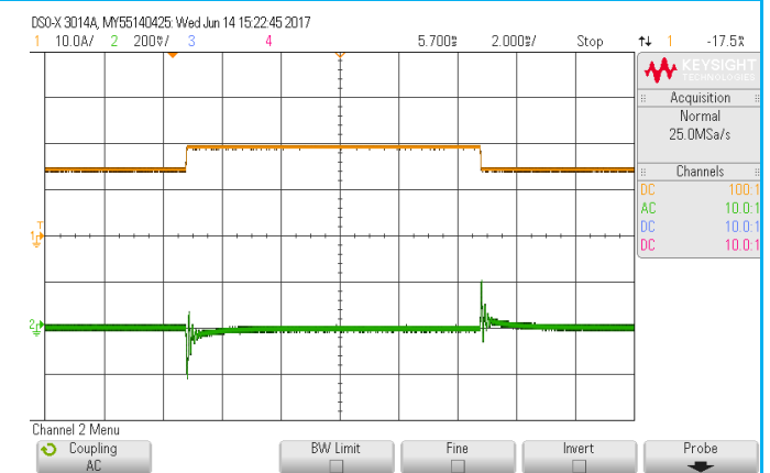
输出电压动态波形 (额定输出, 75%~100%~75% Iout)
