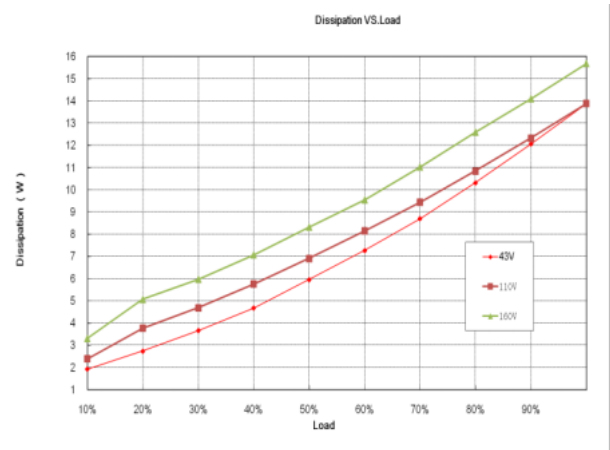
损耗曲线
