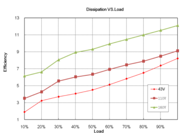
损耗曲线
