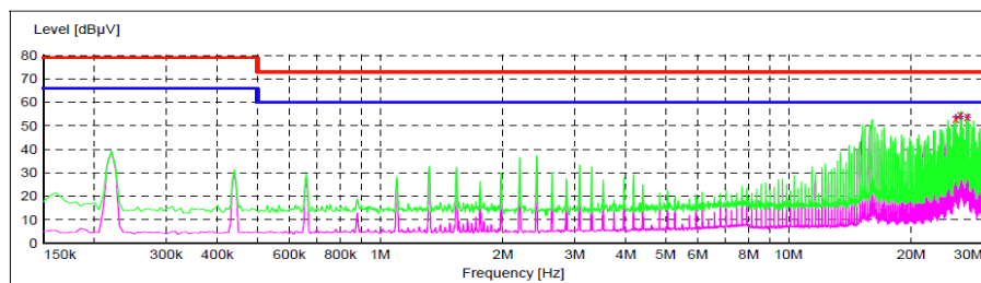
EQ100W-110S24B 模块传导测试结果
