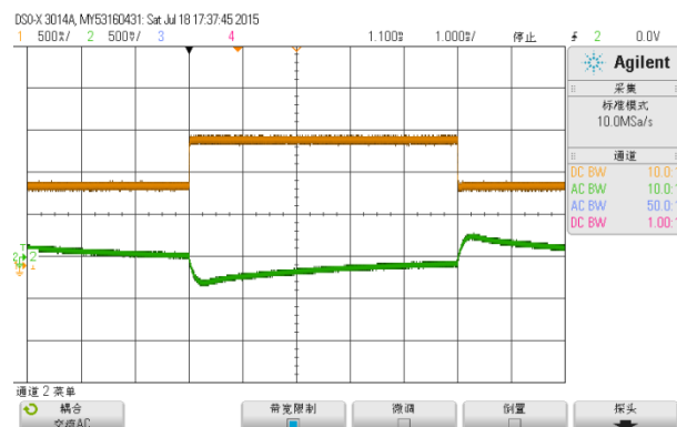
输出电压动态波形 (额定输出, 75%~100%~75% Iout)
