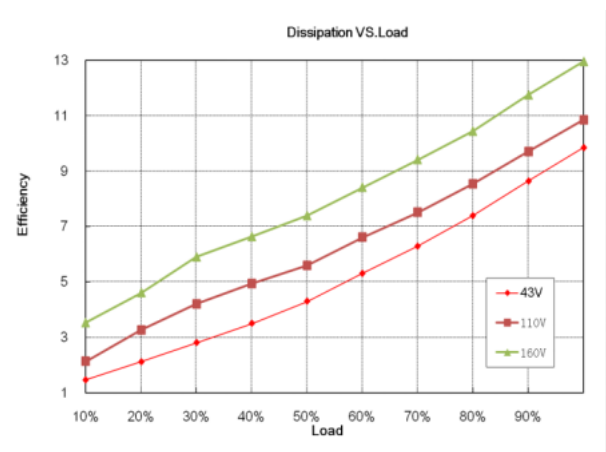
损耗曲线
