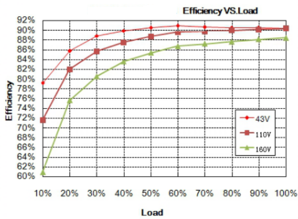
效率曲线
