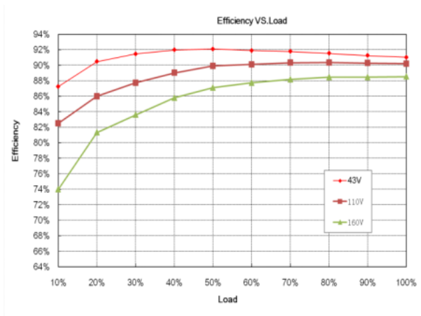
效率曲线
