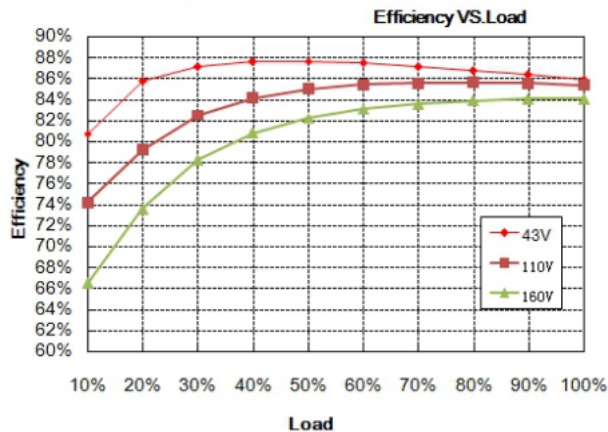
效率曲线
